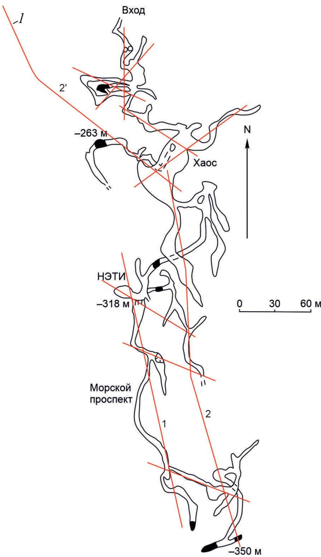
Рис. 10. План пещеры Кёк-Таш. I — разломы и их номера.
