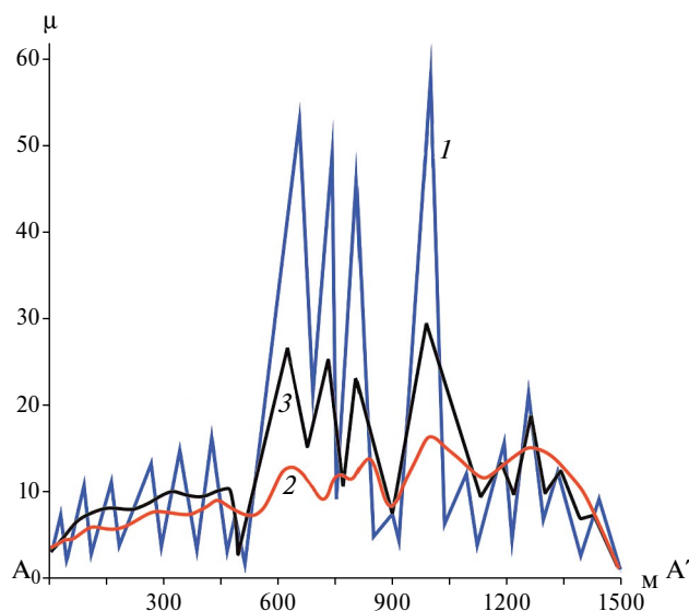
Рис. 5. Осреднение первичных данных по профилю А–А' на участке Дудинская пещера.
