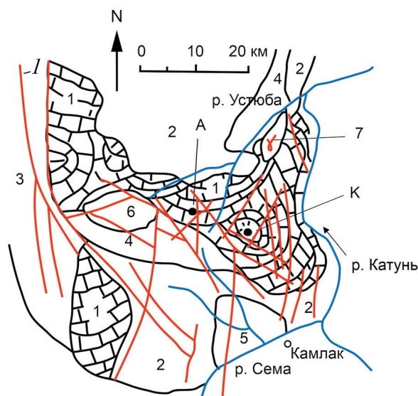
Рис. 8. Геолого-тектоническая схема района пещер Алтайской и Кёк-Таш.
