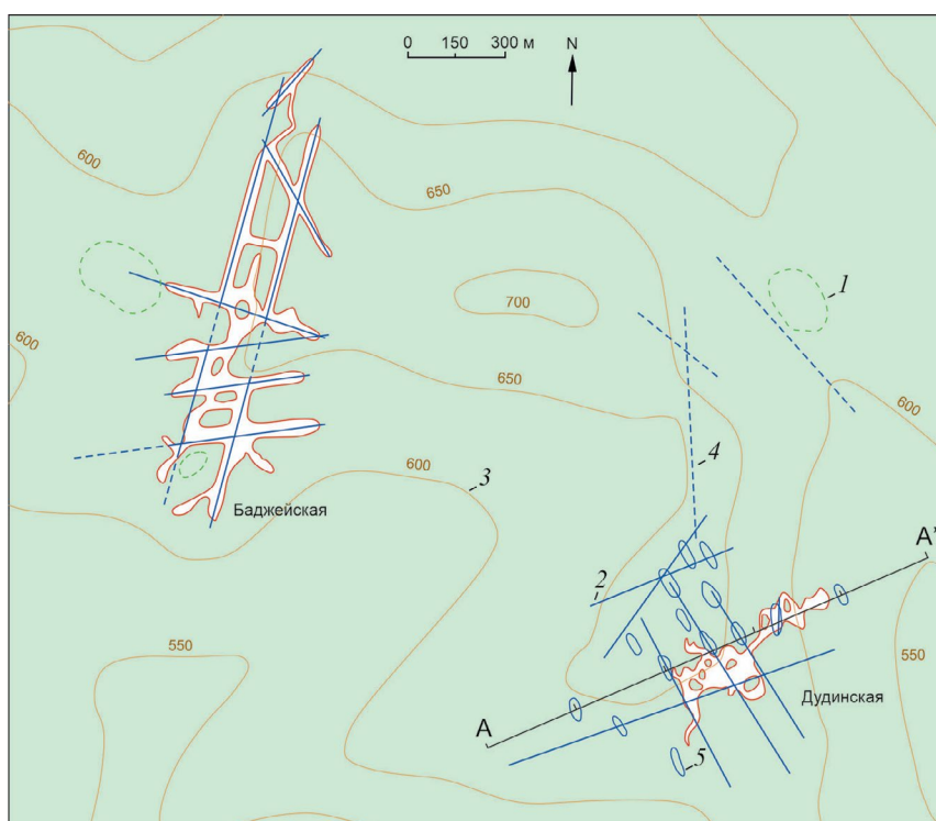
Рис. 4. Выявленные разломы и привязка пещер Баджейская и Дудинская к дневной поверхности. А—А' — профиль измерений трещиноватости; 1 — локальные плато; 2 — разломы; 3 — горизонталы с отметками высот; 4 — предполагаемые разломы; 5 — зоны повышенной плотности трещиноватости; тонирование — массивы пород.
