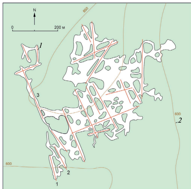
Рис. 7. Разломы, выявленные внутри пещеры Дудинской, и привязка к поверхности.
