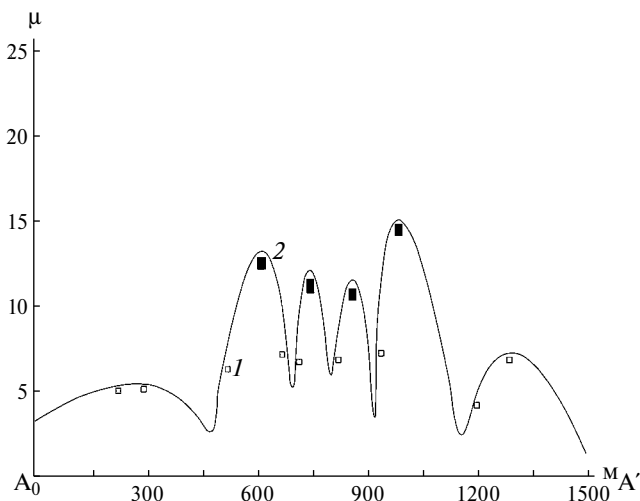
Рис. 6. Спектр распределения плотности трещин по профилю А–А' на участке Дудинская пещера. 1 — зоны дробления; 2 — зоны разломов.
