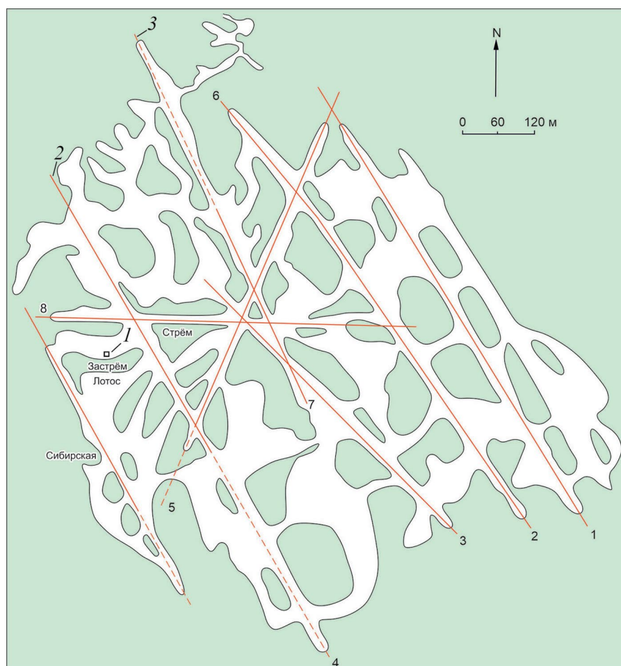
Рис. 2. Схема пещеры Большая Орешная и прослеженные разломы, по которым развита пещера. 1 — площадка геофизических измерений; 2 — разломы, их номера (названия в тексте) и соответствующие им линейные структуры пещеры; 3 — предполагаемые разломы; тонирование — массивы пород.
