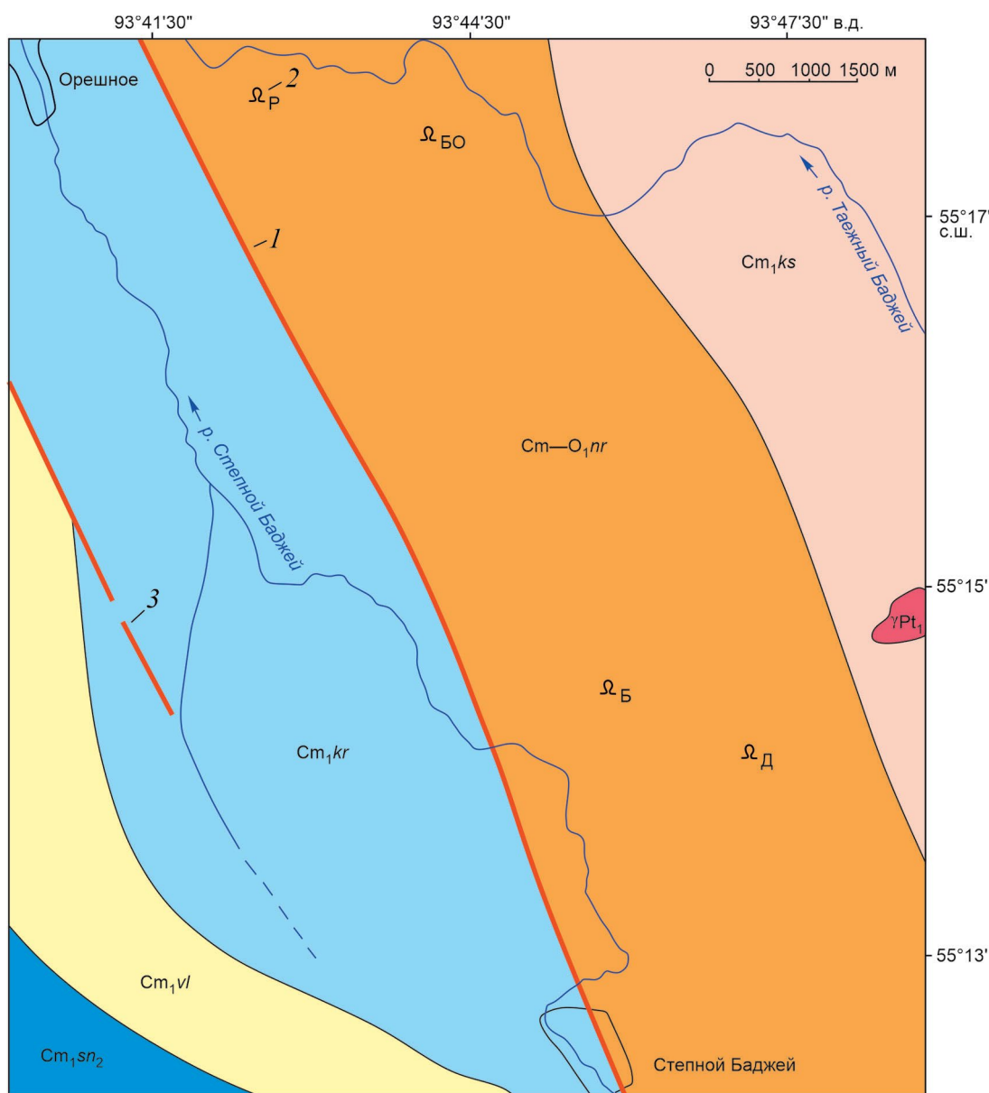
Рис. 1. Геолого-тектоническая схема Баджейского участка.
