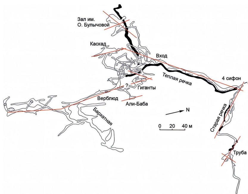
Рис. 9. План пещеры Алтайская. I — разломы.
