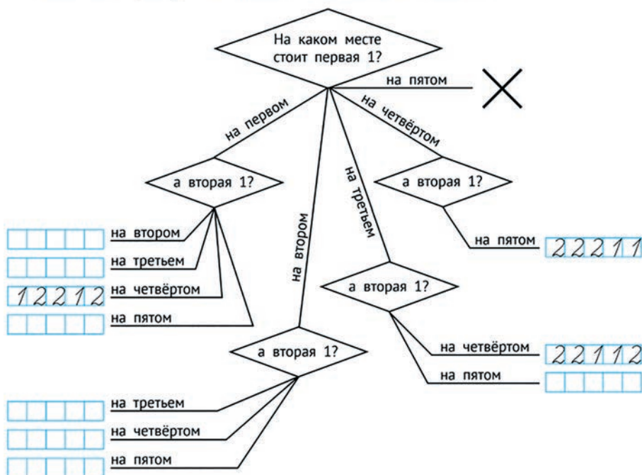
Рис. 28. Задача о цепочках из единиц и двоек.
