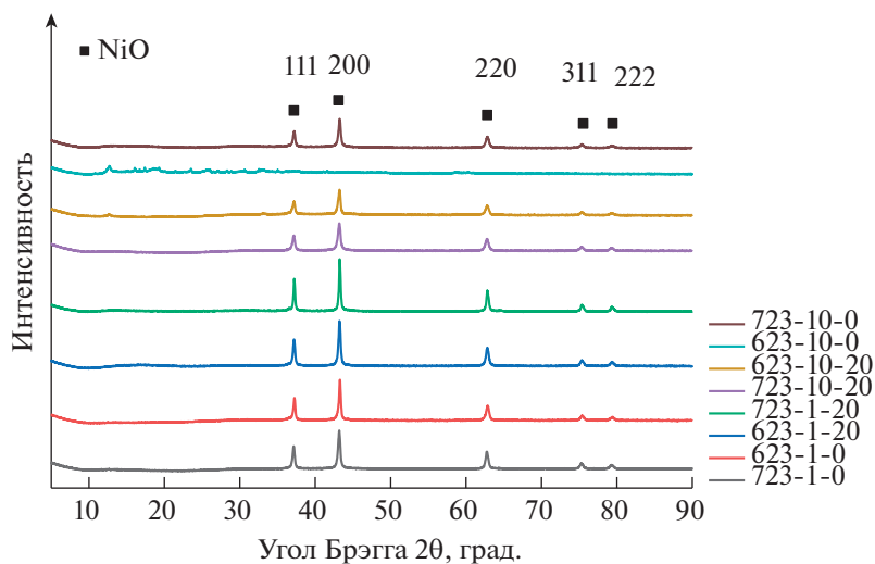
Рис. 4. Дифрактограммы образцов катализатора ( CuK_{\alpha} -излучение, 1.54 Å).
