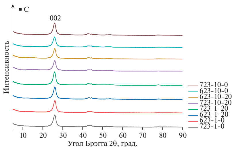
Рис. 5. Дифрактограммы образцов углерода ( \text{CuK}\alpha -излучение, 1.54 Å).
