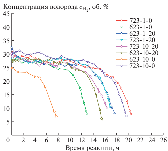
Рис. 3. Зависимость концентрации водорода в процессе каталитической реакции разложения метана при T_p = 823 \text{ К} , p = 1 \text{ атм} .
