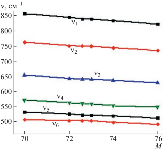
Рис. 2. Зависимости частот \nu пиков фонового поглощения изотопически чистых монокристаллов германия от M — массового числа изотопа для пиков табл. 2.
