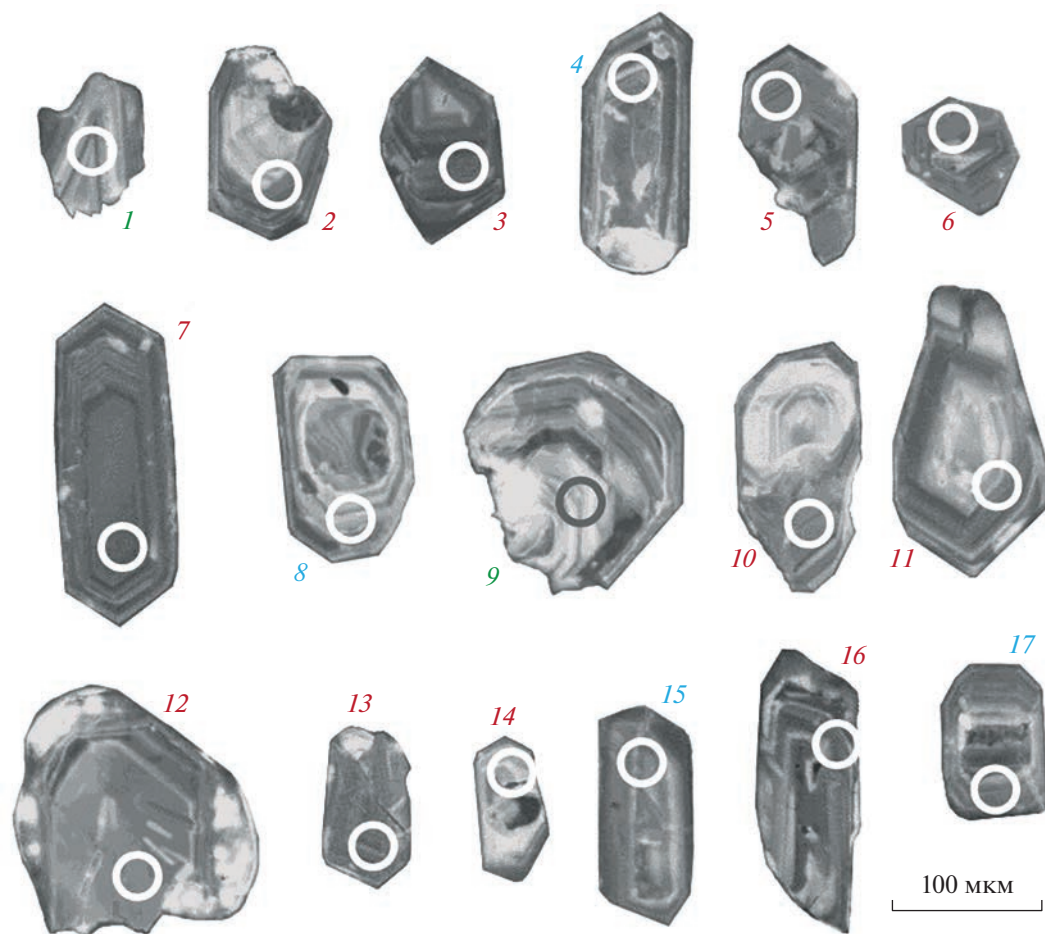
Рис. 3. Катодолюминесцентные изображения кристаллов циркона из гранодиоритов-гранитов Сардаринского (Сарыктинского) массива. Окружностями обозначены точки, где проводилось изотопное датирование, номера точек соответствуют таковым в табл. 2.
