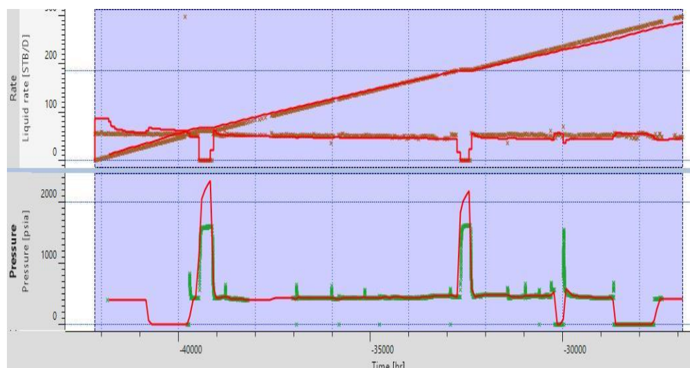
Рис. 2. Обработка данных по истории добычи в модуле Toraze на примере скв. 66 Шершневого месторождения
