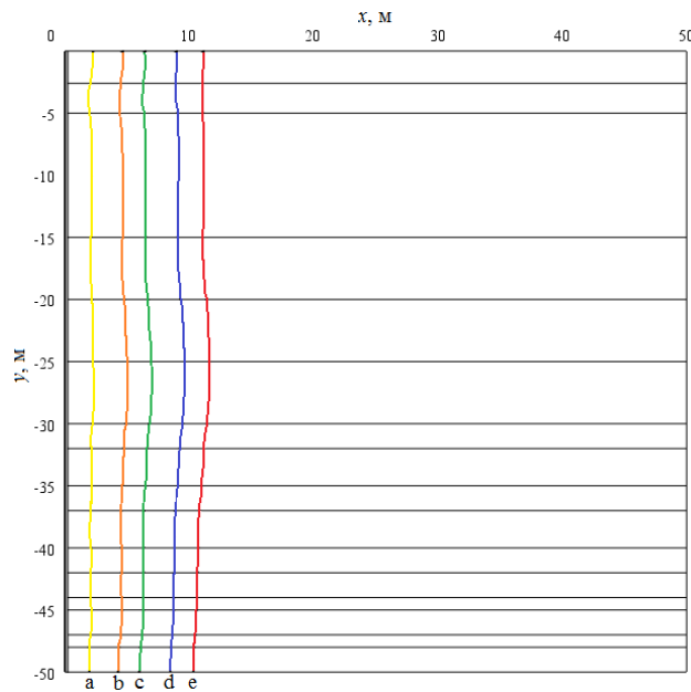
Рис. 5. Изотермические линии 273,15 К в рассматриваемой области решения при T_1=298,15 К: а) 1 год; б) 5 лет; в) 10 лет; д) 20 лет; е) 30 лет
