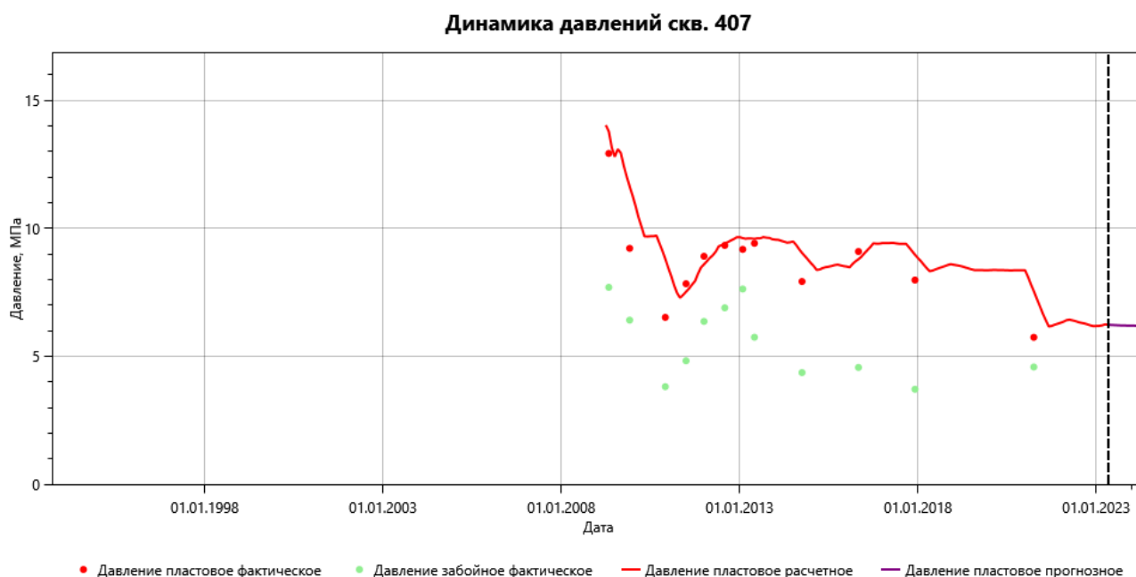
Рис. 7. Результаты определения пластового давления методами машинного обучения в DSA на примере скв. 407 Гагаринского месторождения
