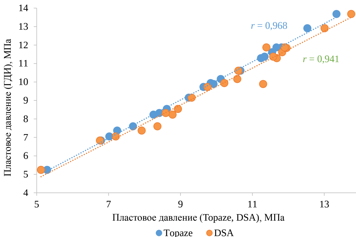
Рис. 4. Сопоставление рассчитанных и фактических пластовых давлений для условий Шершневского месторождения Fig. 4. Comparison of calculated and actual reservoir pressures for the conditions of the Shershnevskoe field
