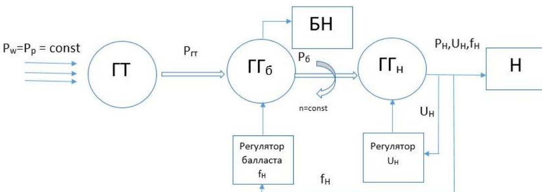
Рис. 3. Генерирующая система с балластным генератором
