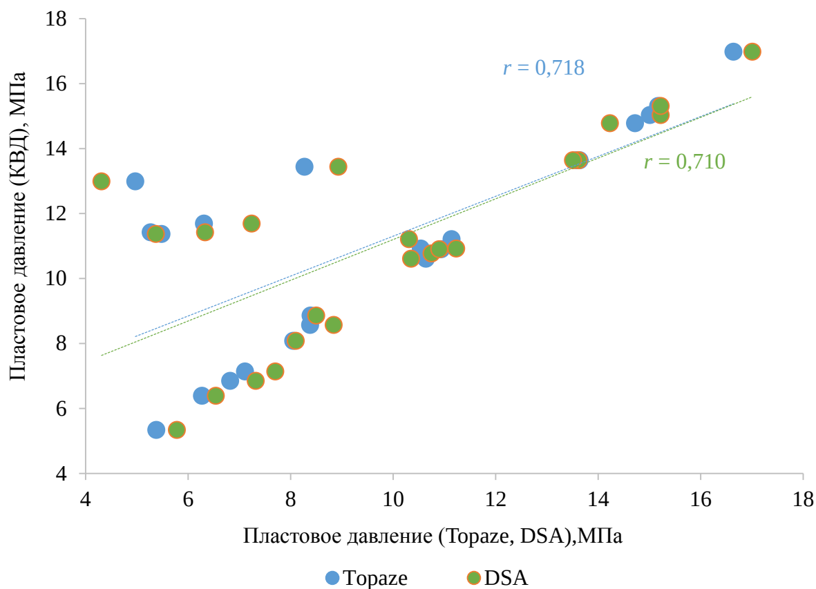
Рис. 6. Сопоставление рассчитанных и фактических пластовых давлений для условий Гагаринского месторождения
