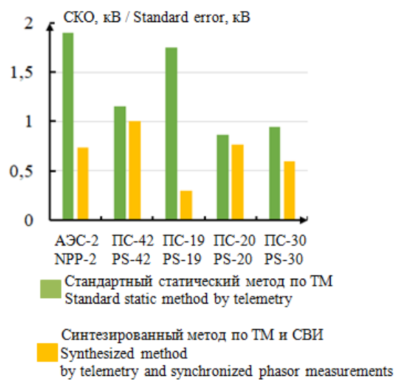
Рис. 4. Распределение среднеквадратичного отклонения напряжения в послеаварийном режиме Fig. 4. Sharing standard voltage deviation in the post emergency state
