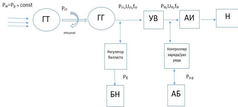
Рис. 9. Структурная схема инверторной микро-ГЭС с автобалластной системой регулирования гидроагрегата и аккумуляторным накопителем электроэнергии
