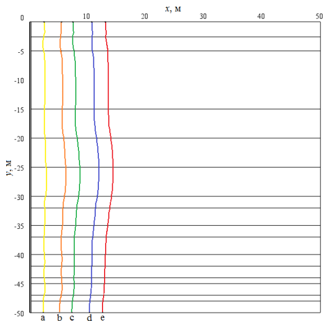
Рис. 4. Изотермические линии 273,15 К в рассматриваемой области решения при T_1=323,15 К: а) 1 год; б) 5 лет; в) 10 лет; д) 20 лет; е) 30 лет
