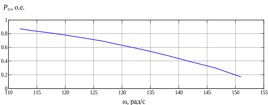
Рис. 8. Зависимость мощности гидрогенератора от угловой скорости вращения Fig. 8. Dependence of the angular rotation speed of the hydrogenerator on active load power
