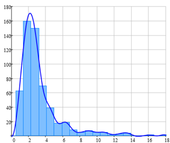
Рис. 8. Пример построения функции распределения частиц по размерам. Слева – изображение, справа – функция распределения частиц по размерам. Непрерывное распределение интерполировалось кубическим сплайном
