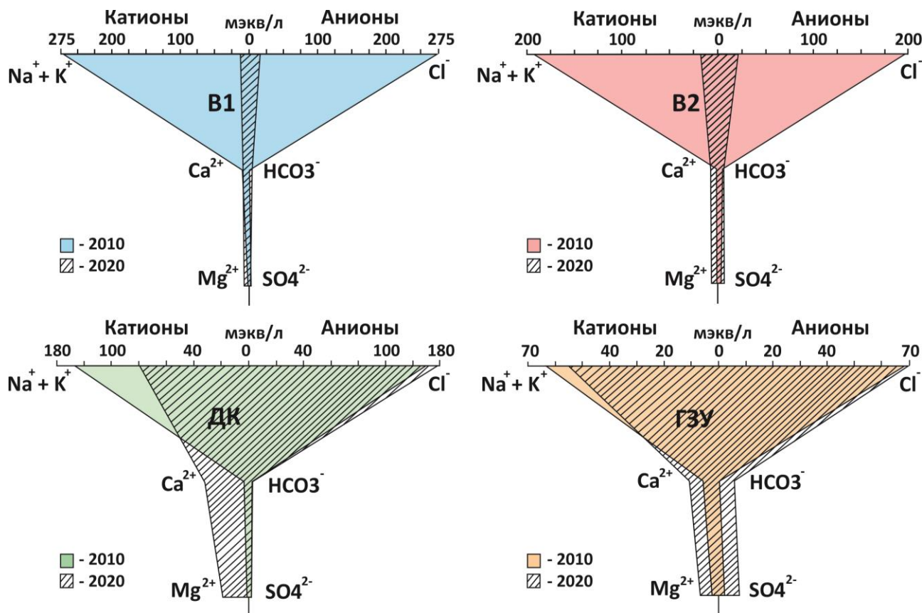
Рис. 2. Диаграммы Стиффа для сточных вод выпуска 1 (B1), выпуска 2 (B2), канавы ГЗУ и дренажной канавы (ДК) в 2010–2020 гг.
