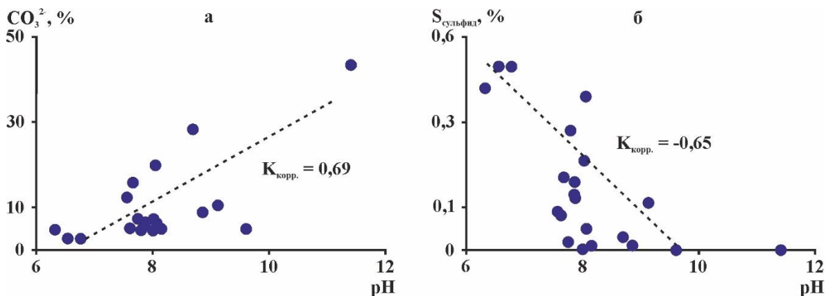
Рис. 3. Связь между \text{pH} в пероксидных растворах и содержаниями \text{CO}_3^{2-} (а) и S_{\text{сульфид}} (б) в породах месторождения Улюк-Бар
