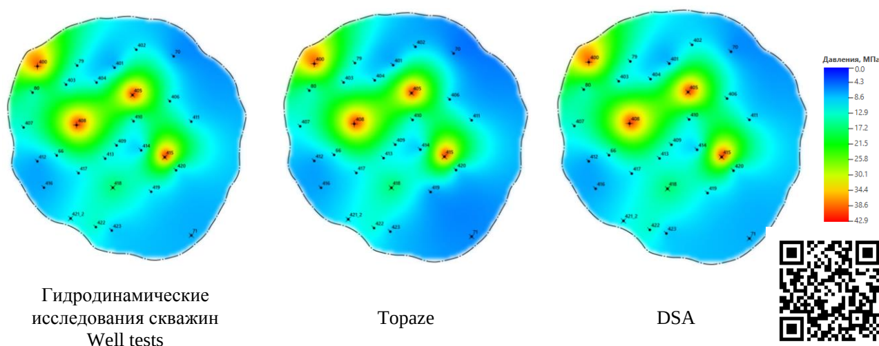
Рис. 3. Карты изобар, построенные для Шершневого месторождения по данным реализации косвенных методов определения пластового давления и ГДИ
