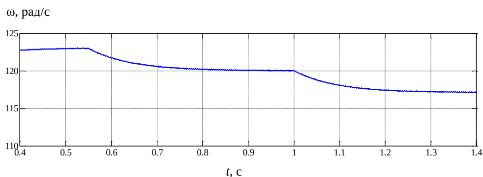
Рис. 7. Переходный процесс изменения скорости вращения при набросе нагрузки инверторной микро-ГЭС Fig. 7. Transient process of changing the angular rotation speed when loading an inverter microelectric power station
