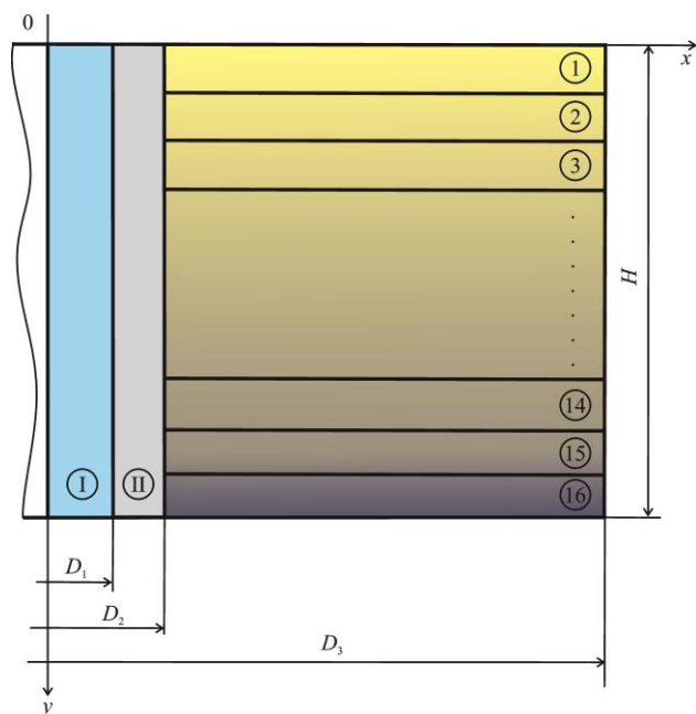
Рис. 1. Схема области решения: I – трубопровод; II – цементные колонны, кондуктор и направления; 1–16 – слои породы/грунта (табл. 1)
