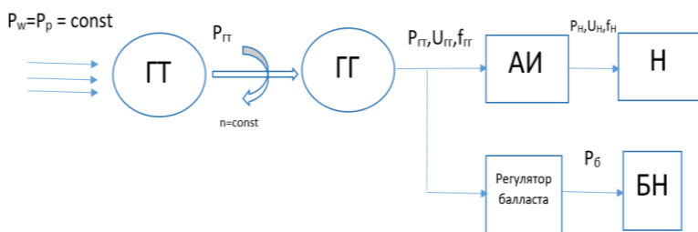
Рис. 5. Структурная схема микро-ГЭС автобалластного типа с инвертором
