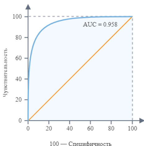
Рис. 1. Метрика AUC-ROC
