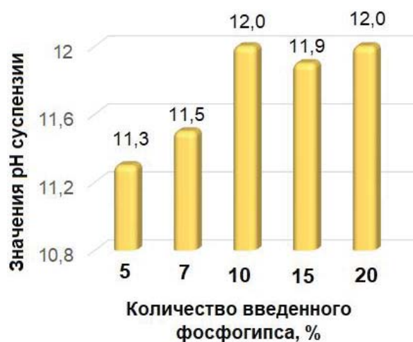
Рис. 4. Значения pH суспензии фосфогипса с различным содержанием реагента
