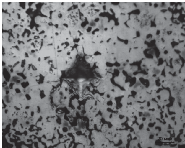
Рис. 8. Отпечаток индентора на поверхности образца при нагрузке 200 г Fig. 8. Indenter imprint on the sample surface at a load of 200 g
