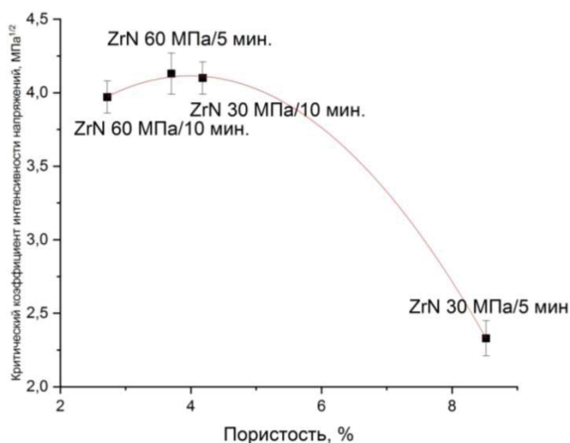
Рис. 9. Зависимость критического коэффициента интенсивности напряжений от пористости Fig. 9. Dependence of the critical stress intensity factor on porosity
