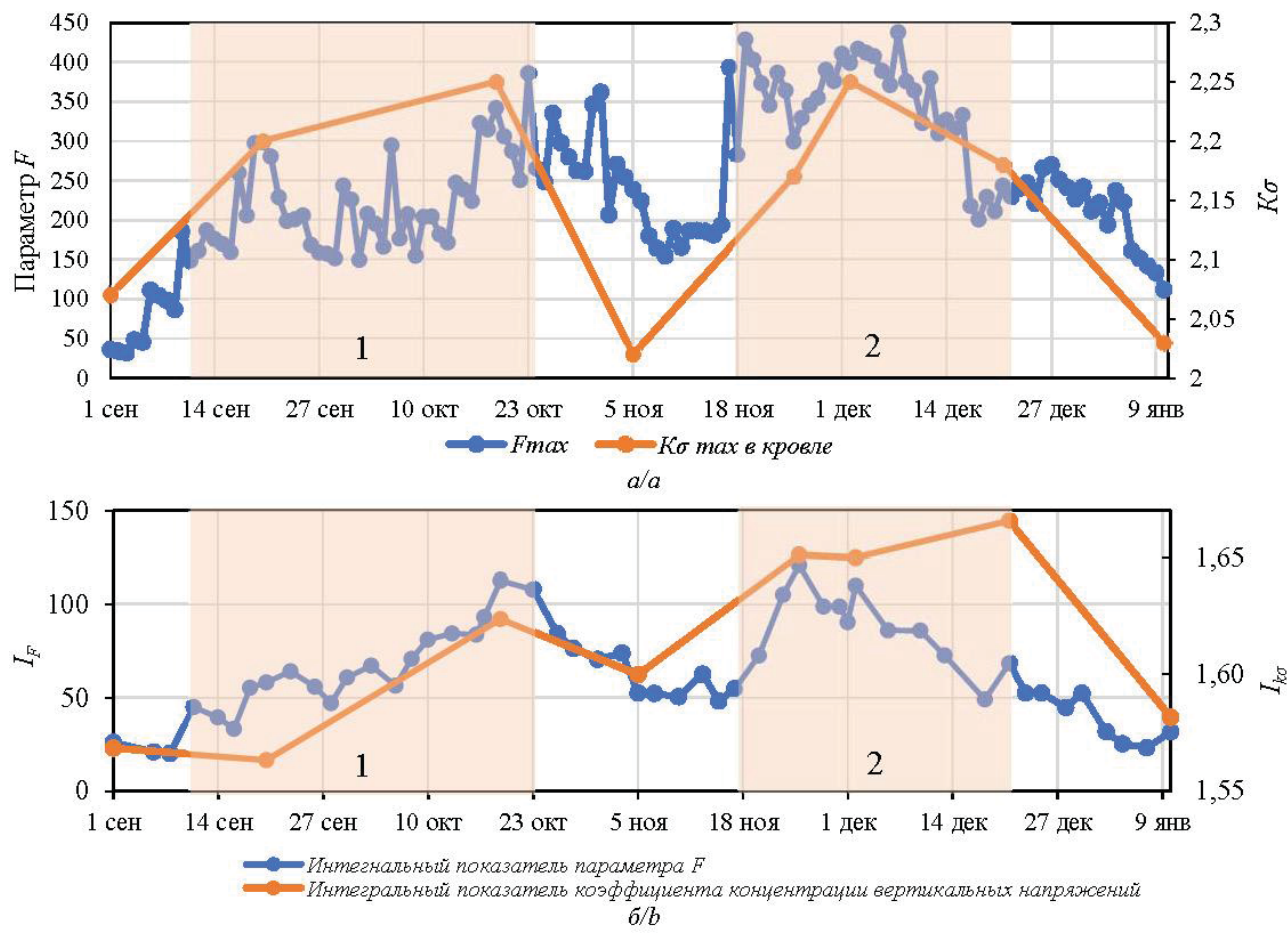
Рис. 1. Графики изменения максимальных значений коэффициента концентрации вертикальных напряжений в кровле пласта Е-5 K_{\sigma-max} кр. и параметра F впереди забоя лавы (а) и интегральных показателей F и K_{\sigma} (б): 1 – перегруз очистным забоем группы тектонических нарушений; 2 – перегруз очистным забоем передовой выработки и тектонических нарушений
