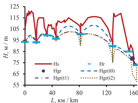
Рис. 4. Профиль АР–ОР (рис. 1, б) и уровни подземных вод в голоцене: H_s – поверхность водосбора или дна рек; H_r – современный среднегодовое значение уровня речных вод; H_{gr} – современный среднегодовое значение уровня воды в скважине 63р в с. Мельниково; H_{gr}(t_0) – расчетный среднегодовой уровень подземных вод в среднем за 1967–2005 гг.; H_{gr}(t_1) – расчетный уровень подземных вод при условии, что все болота низинного типа, а их площадь в 1,7 раз больше, чем в настоящее время (ориентировочно 1,5...2,0 тыс. лет назад); H_{gr}(t_2) – расчетный уровень подземных вод при условии, что все болота низинного типа с глубиной не более 0,3 м, а их площадь в 2 раза меньше, чем в настоящее время (ориентировочно 4 тыс. лет назад)
