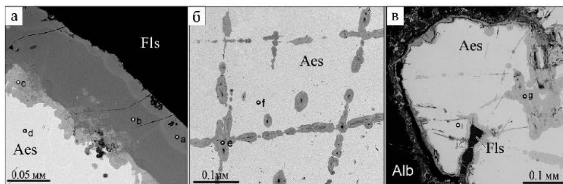
Рис. 6. Округлые зональные текстуры метасоматических изменений в эшините (участки d, f, i).
