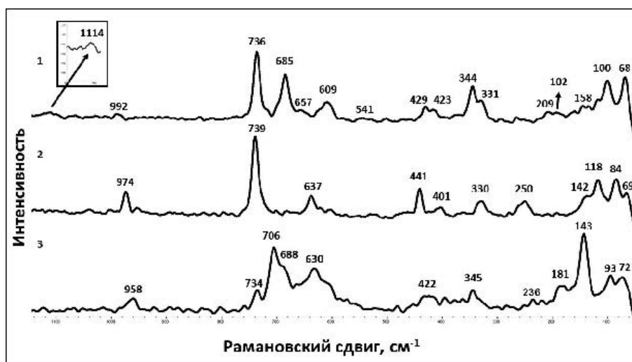
Рис. 6. КР спектры гипергенных минералов Te месторождения Приозёрное.
