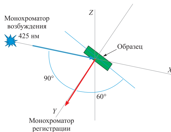
Рис. 1. Геометрия эксперимента.
