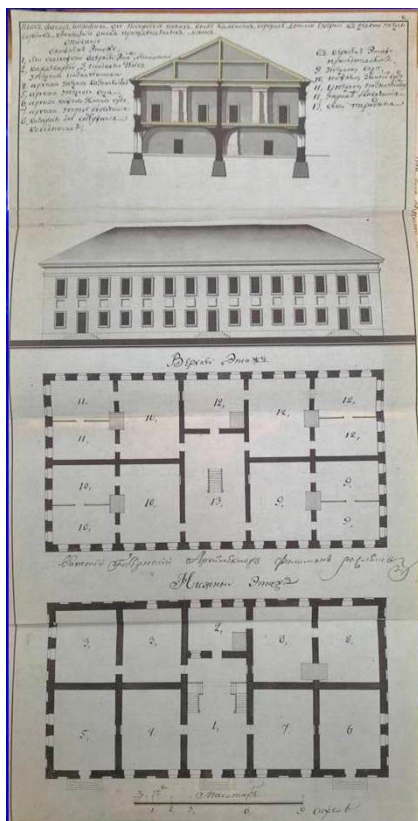
Рис. 2. План фасада каменного корпуса присутственных мест в уездных городах (1 этаж, помещение № 3 — кладовая для хранения денег). Архитектор Ф. М. Росляков. 1798 год [ЦГАКО, ф. 176, оп. 6, д. 10, л. 163а]
