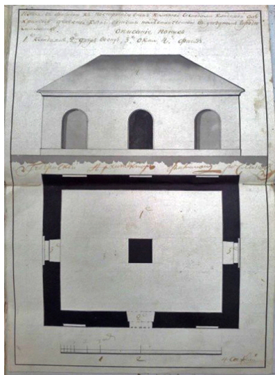
Рис. 1. План с фасадом каменной кладовой для хранения денежной казны в уездном городе Малмыже. Архитектор Ф. М. Росляков. 1796 год [ЦГАКО, ф. 176, оп. 6, д. 10, л. 39 а]
