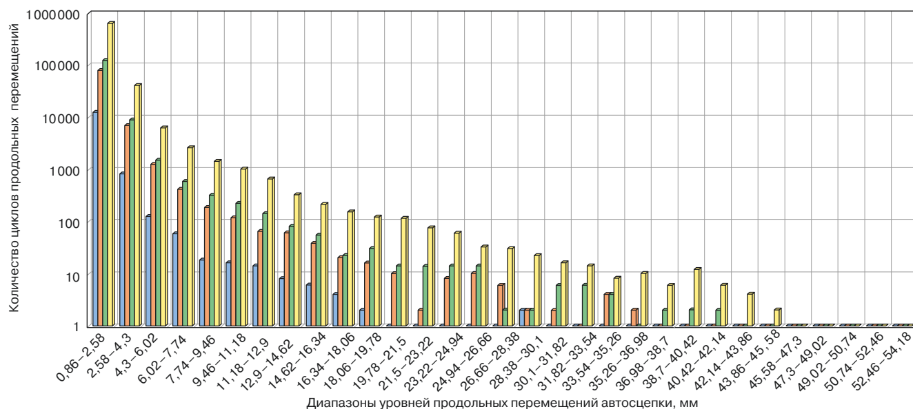
Рис. 10. Статистическая гистограмма распределения размахов продольных перемещений автосцепки относительно кузова для различных участков пути по всему маршруту следования, на 10 тыс. км пробега:
