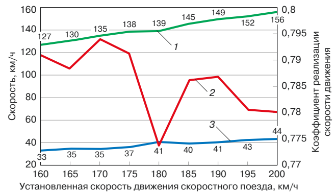
Рис. 3. Изменение фактической скорости и коэффициента реализации скорости: 1 — фактическая маршрутная скорость; 2 — коэффициент реализации скорости движения; 3 — разность установленной и фактической маршрутной скорости
