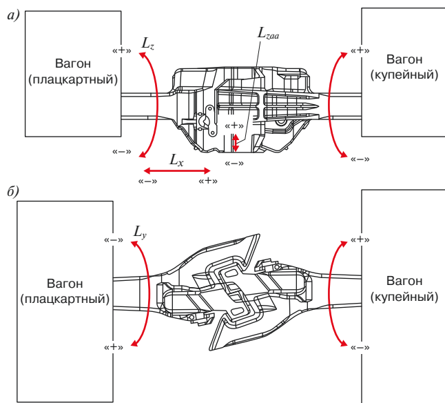
Рис. 1. Регистрируемые при испытаниях процессы (кузова вагонов показаны условно) вид сбоку (а), вид сверху (б): L_x — линейные перемещения автосцепки относительно кузова в продольном направлении; L_y — угловые перемещения автосцепки относительно кузова в горизонтальной плоскости; L_z — угловые перемещения автосцепки относительно кузова в вертикальной плоскости; L_{zda} — взаимные относительные линейные перемещения автосцепок в вертикальном направлении
