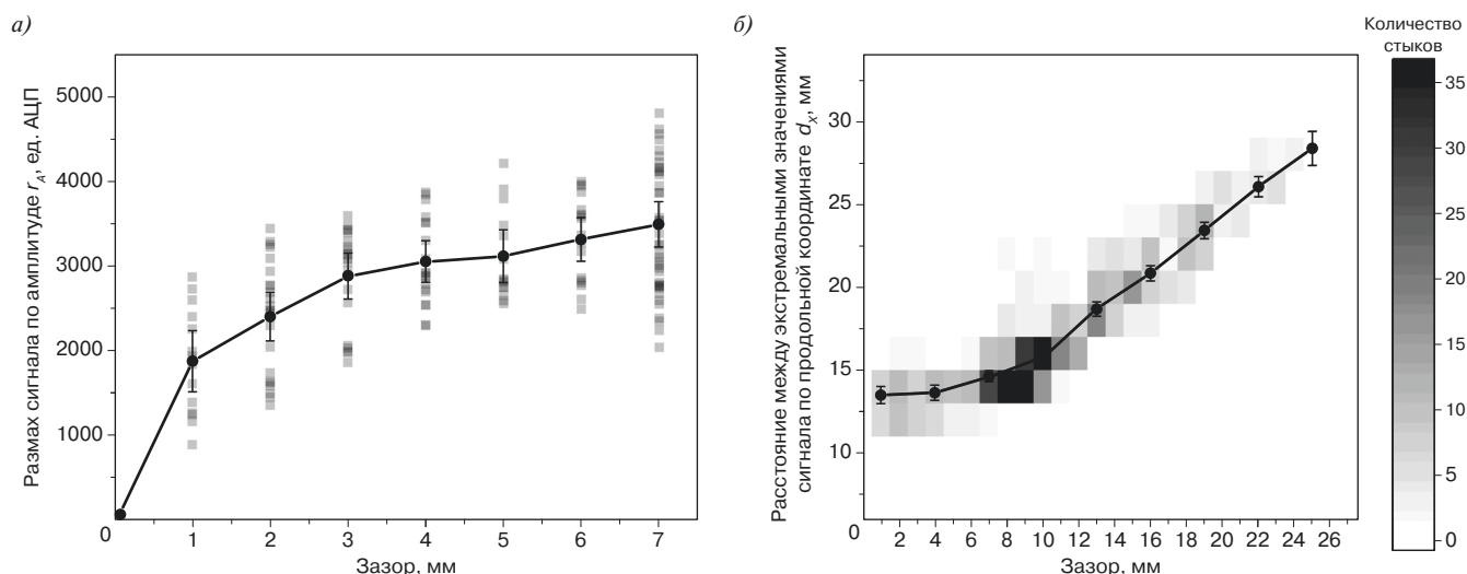
Рис. 4. Зависимости размаха по амплитуде r_A (а) и расстояния между экстремумами d_X (б) сигнала от величины зазора болтового стыка, полученные по данным эксперимента [3]
