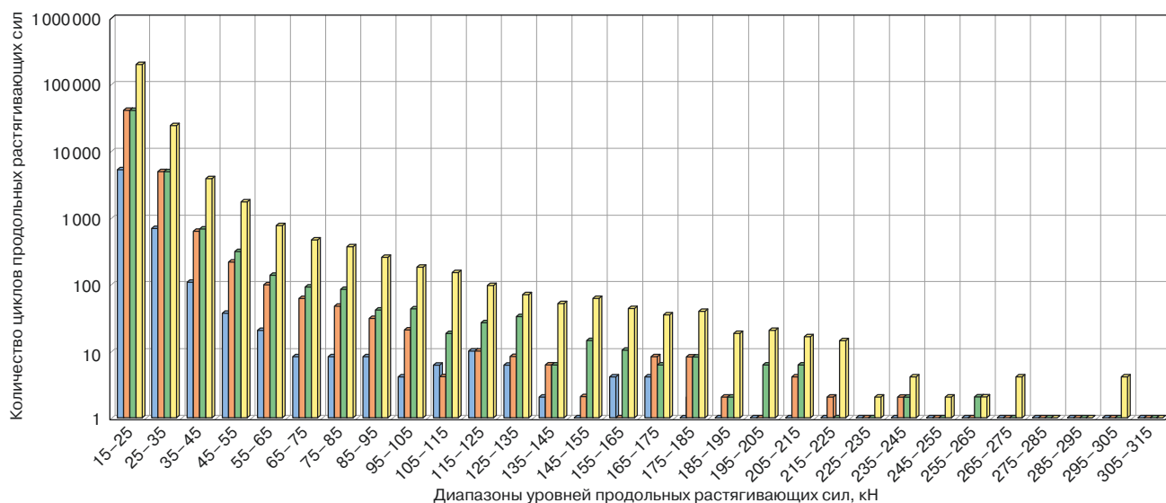
Рис. 5. Статистическая гистограмма распределения размахов продольных растягивающих сил в автосцепке для различных участков пути по всему маршруту следования, на 10 тыс. км пробега:
