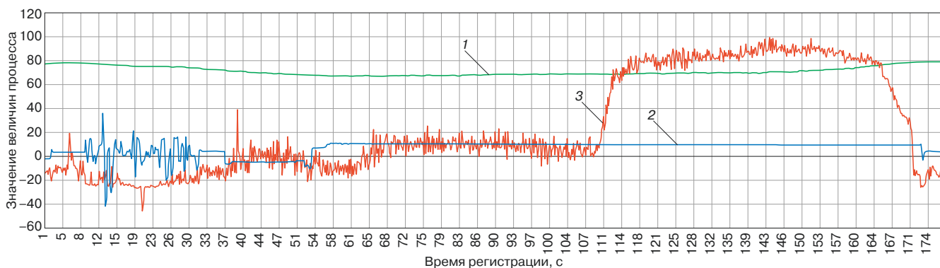
Рис. 3. Пример записи процессов продольной силы и относительных вертикальных перемещений автосцепок для случая движения вагона в голове состава:
