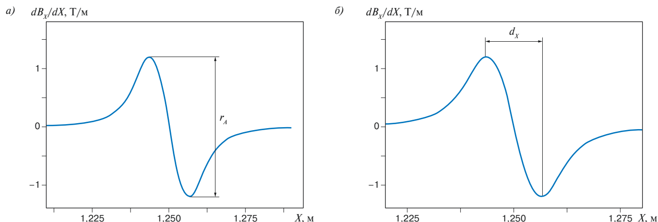
Рис. 3. Информационные параметры импульса от стыкового зазора (поз. 1 на рис. 2): а — размах по амплитуде; б — расстояние между экстремумами
