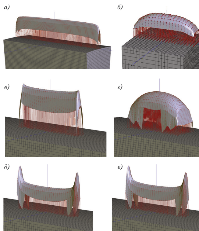
Рис. 4. Распределение давлений на поверхностях контакта образцов: а — цилиндрический образец, D=40 мм, B=8 мм, решение в упругой постановке, P=880 Н, p_0=1000 МПа; б — цилиндрический образец, D=40 мм, B=3 мм, решение в упругопластической постановке, P=880 Н, p_0=1000 МПа; в — образец с буртиком, h=3 мм, b=3 мм, решение в упругой постановке, P=880 Н, p_0=1000 МПа; г — образец с буртиком, h=3 мм, b=3 мм, решение в упругопластической постановке, P=3600 Н, p_0=1420 МПа; д — образец с фасками, снятыми под углами 30^\circ , b=3 мм, решение в упругой постановке, P=1000 Н, p_0=1000 МПа; е — образец с фасками, снятыми под углами 45^\circ , b=3 мм, решение в упругой постановке, P=1000 Н, p_0=1000 МПа
