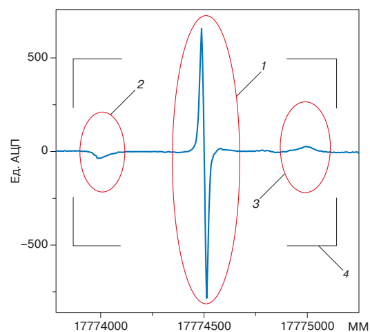
Рис. 2. Фрагмент дефектограммы участка рельса длиной около 1,5 м: 1 — сигнал магнитного датчика от стыкового зазора; 2, 3 — импульсы от концов стыковых накладок; 4 — автоматически распознанная программой зона болтового стыка
