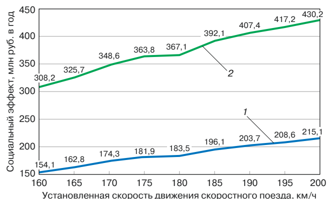
Рис. 4. Изменение социального эффекта: 1 — 5-вагонный состав; 2 — 10-вагонный состав
