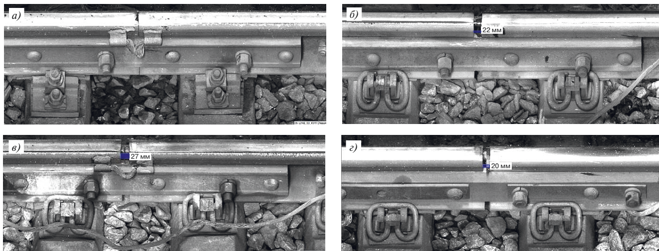
Рис. 5. Болтовые стыки с минимальным (а), номинальным (б) и максимальным (в) зазором; г — изолирующий стык с недопустимо большим (20 мм) зазором. Значения отображаются при наведении курсора мыши на кадрах
