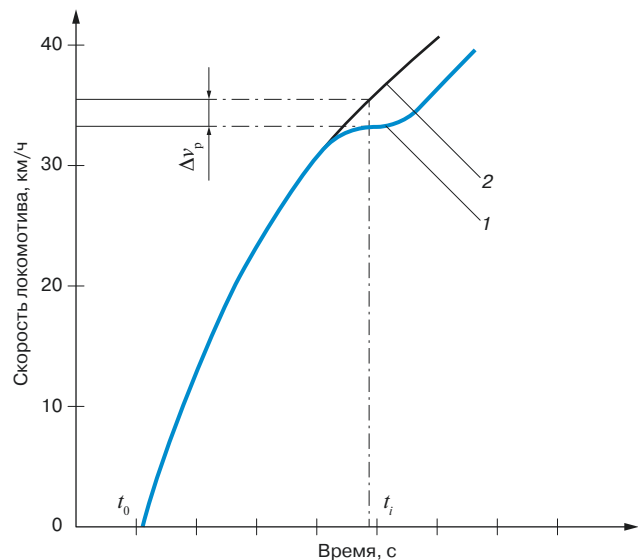
Рис. 4. Определение силы сопротивления движению на основе кривой скорости: 1 — фактическая скоростная кривая; 2 — расчетная скоростная кривая
