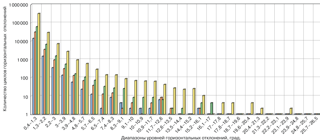
Рис. 8. Статистическая гистограмма распределения размахов горизонтальных угловых отклонений автосцепки для различных участков пути по всему маршруту следования, на 10 тыс. км пробега:
