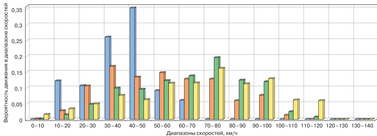
Рис. 2. Гистограмма распределения скоростей движения вагона в составе поезда для различных участков пути по маршруту следования Анапа — Санкт-Петербург:
