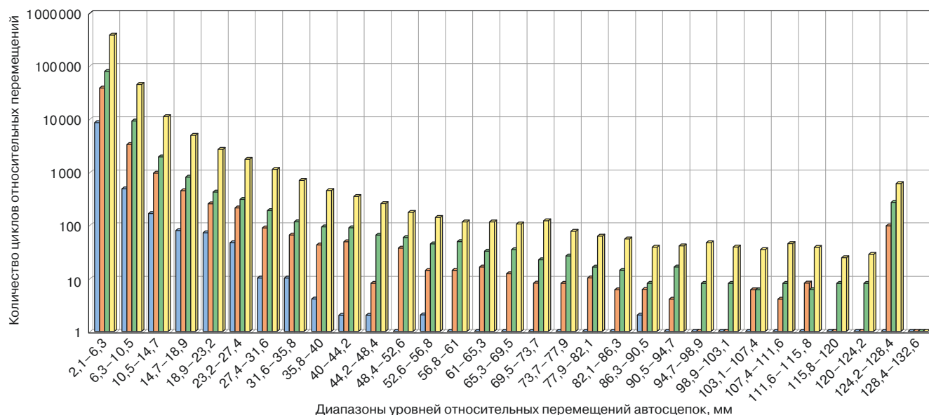
Рис. 9. Статистическая гистограмма размахов относительных перемещений автосцепок для различных участков пути по всему маршруту следования, на 10 тыс. км пробега:
