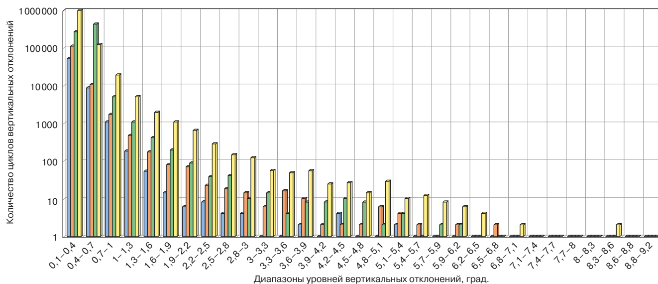
Рис. 7. Статистическая гистограмма распределения размахов вертикальных угловых отклонений автосцепки для различных участков пути по всему маршруту следования, на 10 тыс. км пробега:
