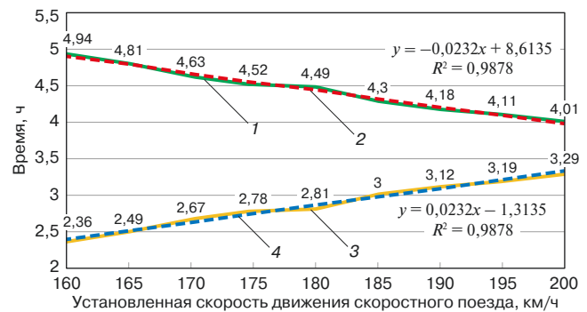
Рис. 2. Изменение параметров проезда: 1 — время в пути; 2 — линейная (время в пути); 3 — экономия времени в пути; 4 — линейная (экономия времени в пути)
