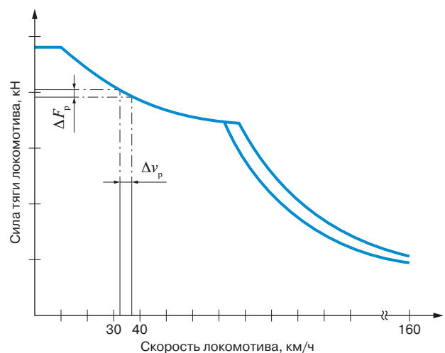
Рис. 5. Условное отображение тяговой характеристики локомотива ЭП20 с конструкционной скоростью 160 км/ч
