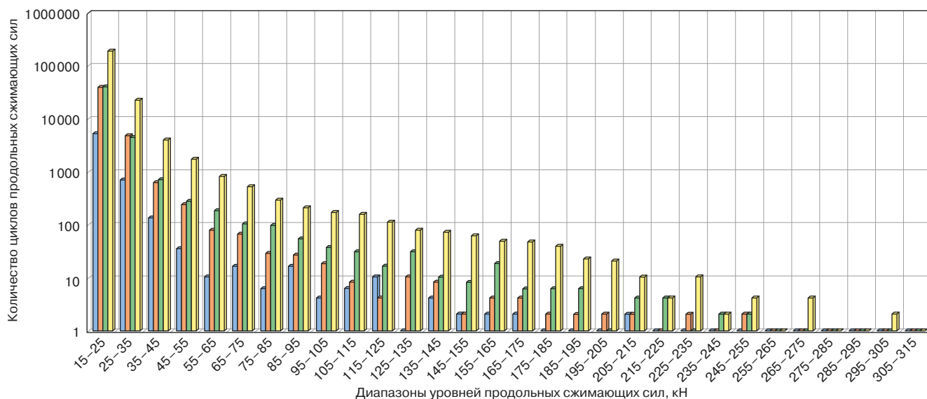
Рис. 6. Статистическая гистограмма распределения размахов продольных сжимающих сил в автосцепке для различных участков пути по всему маршруту следования, на 10 тыс. км пробега:
