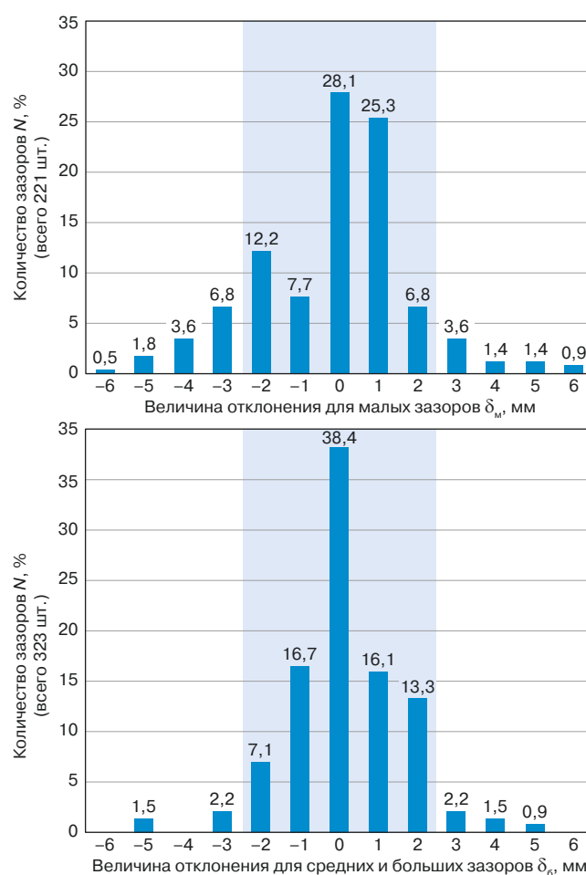
Рис. 8. Отклонения величины стыковых зазоров, определенных по магнитному методу и по видеокадрам для: а — малых (8 мм и менее); б — средних и больших зазоров (9 мм и более)
