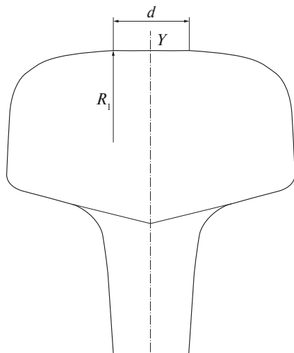
Рис. 6. Параметры контроля профиля рельса
