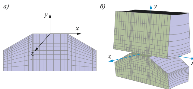
Рис. 8. Конечно-элементная модель:
