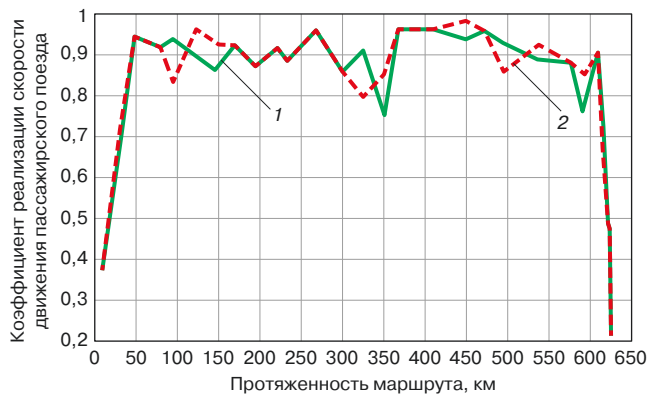
Рис. 1. Изменение коэффициента реализации скорости движения пассажирского поезда по маршруту О—Н: 1 — четное направление; 2 — нечетное направление
