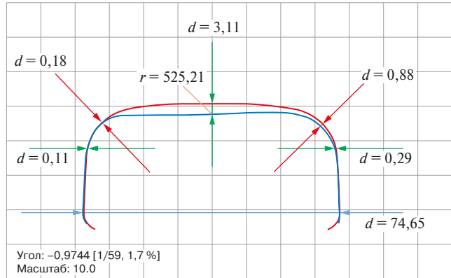
Рис. 8. Поперечный профиль головки рельса внутренней нити кривой радиуса 300 м после пропуска тоннажа 100 млн т брутто Fig. 8. Transverse profile of the rail head of the inner thread of the curve of radius 300 m after handling a tonnage of 100 million gross tons
