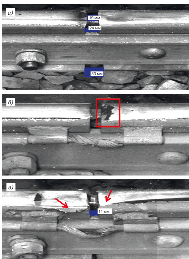
Рис. 6. Стыки с нарушениями: наплыв металла и косой срез торцов рельсов (а), выкрашивание поверхности катания (б), смятия концов рельсов (в)
