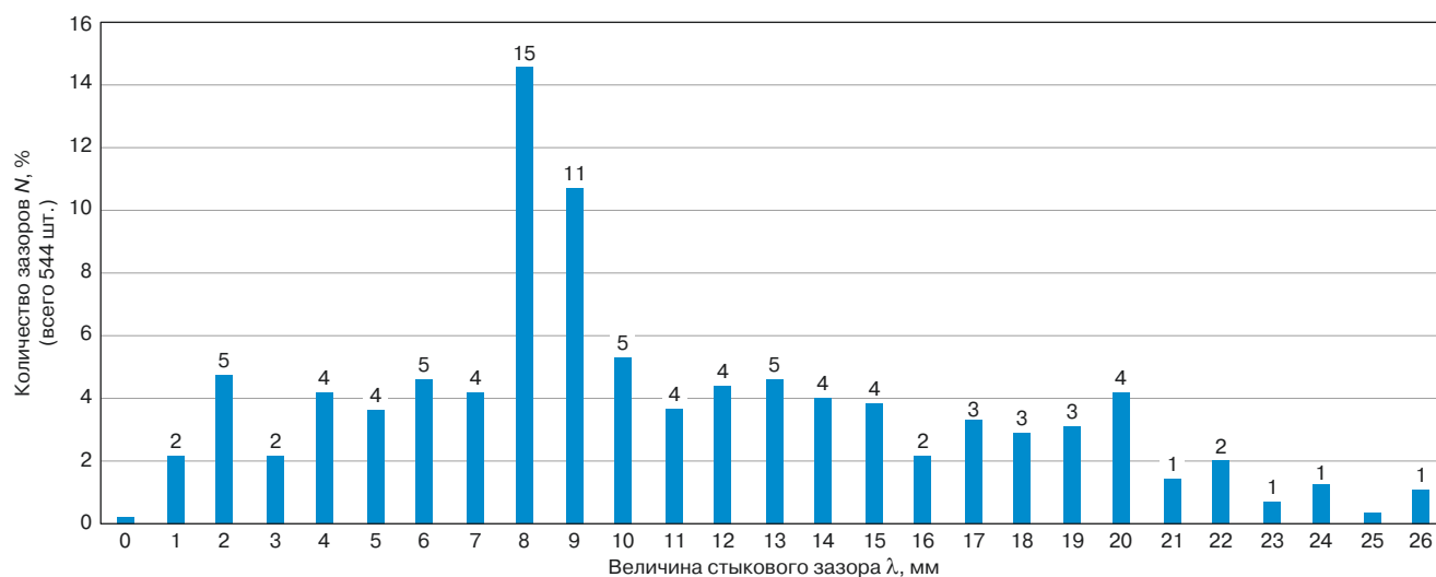
Рис. 7. Распределение величин стыковых зазоров на рассматриваемых участках пути
