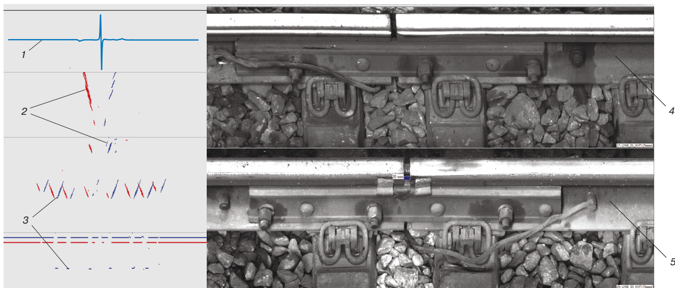
Рис. 1. Отображение сигналов магнитного метода (1), ультразвукового многоканального метода от торцов рельсов (2) и от болтовых отверстий (3), двухракурсного визуального метода изнутри колеи (4) и снаружи (5) в диагностическом комплексе неразрушающего контроля рельсов
