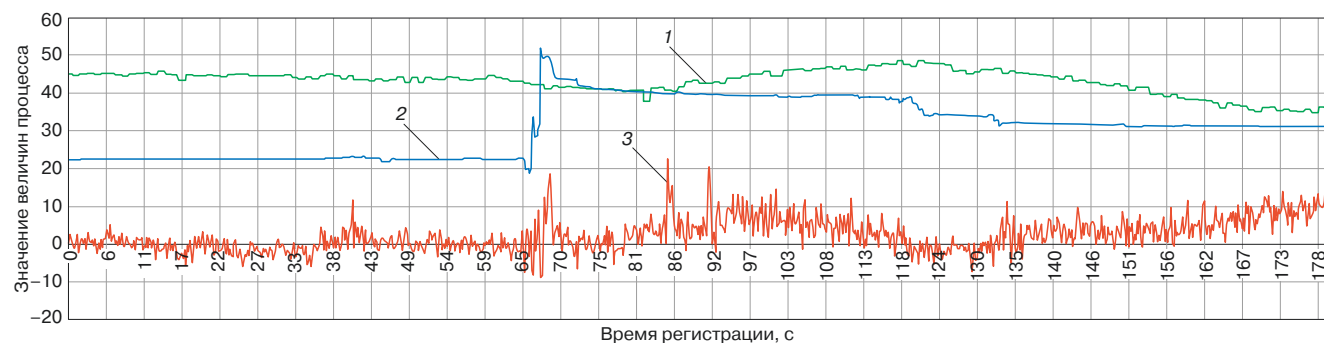
Рис. 4. Пример записи процессов продольной силы и относительных вертикальных перемещений автосцепок для случая движения вагона в хвосте состава:
