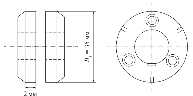
Рис. 2. Составной образец [9, 10]
