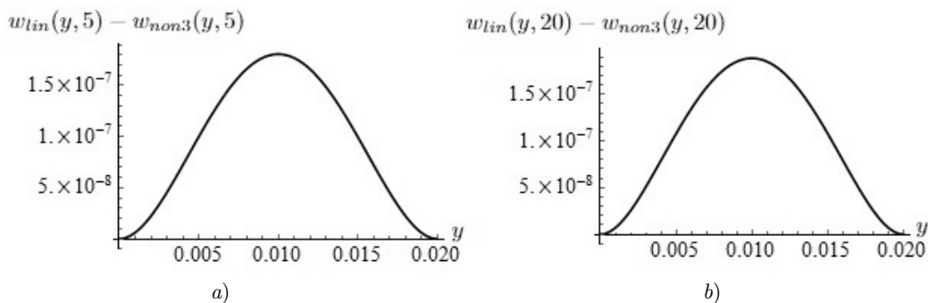
Рис. 6.5. Отличие деформации пластины в моделях (2.9) и (2.12) в моменты времени: а) t = 5 ; б) t = 20
