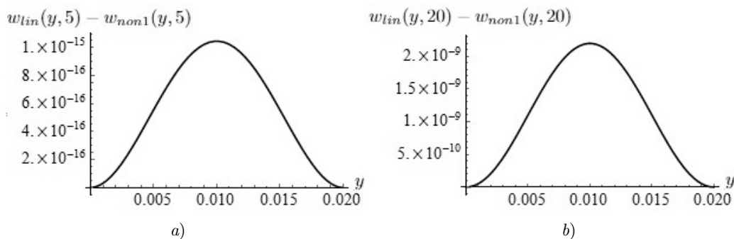
Рис. 6.3. Отличие деформации пластины в моделях (2.9) и (2.10) в моменты времени: а) t = 5 ; б) t = 20
