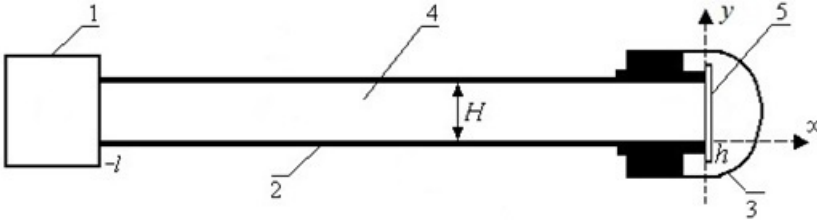
Рис. 3.1. Трубопровод с датчиком
