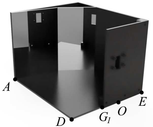
Рисунок 4. 3D-модель катоптрической системы внутри короба с частично прозрачной стороной DE
