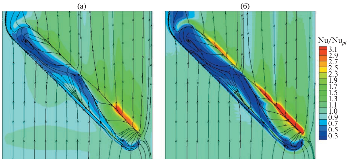
Рис. 2. Рассчитанные поля относительных чисел Нуссельта Nu/Nu_{pl} с нанесенными линиями растекания на контрольном участке структурированной стенки канала при задании граничных условий q = \text{const} (а) и T = \text{const} (б).
