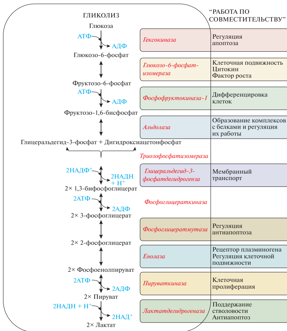
Рис. 1. Мультифункциональность ферментов гликолиза.
