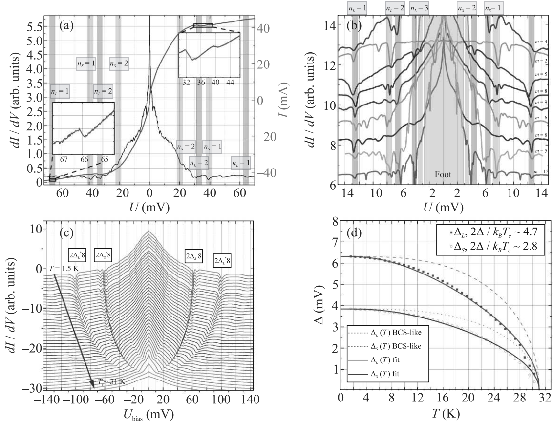
Рис. 2. (Цветной онлайн) (a) – ВАХ и дифференциальная проводимость, измеренные модуляционным методом для одного из контактов. На вставках приведены увеличенные участки ВАХ, содержащие SGS. Вертикальными полосами помечены SGS, содержащие по два андреевских рефлекса. Красным и синим цветами обозначены SGS для большой и малой щели соответственно. (b) – Подборка характеристик дифференциальных проводимостей для разных контактов, нормированными на количество последовательно включенных контактов в стопке – m . (c) – Температурная эволюция дифференциальной проводимости для контакт с m = 8 в температурном диапазоне от 1.5 до 31.5 К с шагом 0.7 К. (d) – Извлеченные из данных панели (c) температурные зависимости большой и малой щели, а пунктирными линиями приведены БКШ-подобные зависимости, а сплошной линией – аппроксимация зависимостью по формуле (7)
