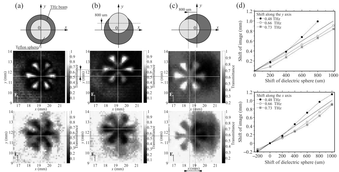
Рис. 4. (Цветной онлайн) Изображения структуры “звезды Сименса” на \text{SiO}_2 подложке, полученные при помощи ПТФЕ сферы диаметром 2.3 мм, размещенной в ТГц пучке. Слева направо: (a) – диэлектрическая сфера расположена в центре перетяжки гауссова ТГц пучка; (b) – положение сферы смещенно на 800 мкм ( 0.35d ) вдоль оси y относительно центра перетяжки гауссова ТГц пучка; (c) – положение сферы смещенно на 800 мкм ( 0.35d ) вдоль оси x относительно центра перетяжки гауссова ТГц пучка. Размер изображений составляет 4 \times 4 мм. Шаг сканирования вдоль осей x и y выбирался равным 102 мкм, расстояние между поверхностью сферы и образцом составляло 200 мкм. (d) – Смещение центра “звезды Сименса” ( \delta_{\text{image}} ) в зависимости от величины смещения ПТФЕ сферы ( \delta_{\text{sphere}} ) и частоты f . Верхний график соответствует \delta_{\text{sphere}} \parallel E , нижний \delta_{\text{sphere}} \perp E . Синяя кривая на графиках соответствует условию \delta_{\text{image}} = \delta_{\text{sphere}}
