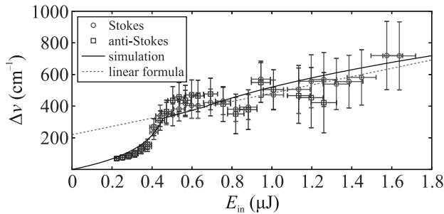
Рис. 5. (Цветной онлайн) Расчетная (сплошная линия) и экспериментальная (точки) зависимости ширины спектра лазерного импульса, прошедшего через образец плавленого кварца, от энергии импульса накачки. Пунктирная линия соответствует наклону для линейного режима
