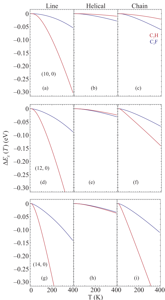
Рис. 3. (Цветной онлайн) \Delta E_g(T) для трубок (10, 0) – (a)–(c); (12, 0) – (d)–(f) и (14, 0) – (g)–(i). Красная линия соответствует структурам C_2H , синяя – C_2F . Графики расположены слева направо в порядке “линия”, “спираль”, “цепочка”
