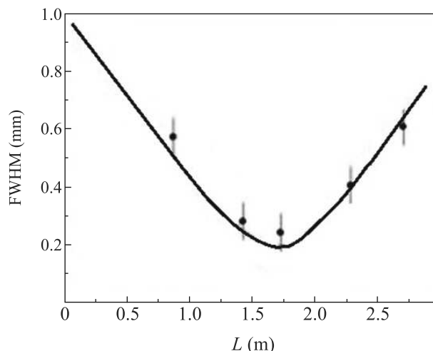
Рис. 2. Огибающая пучка (размер пучка в зависимости от расстояния, отсчитываемого от кристалла). Точки – эксперимент. Кривая – расчет для реальных условий с учетом рассеяния на воздухе и эмульсиях
