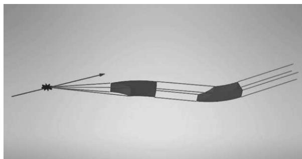
Рис. 3. (Цветной онлайн) Двухкристальная оптическая схема для формирования аксиально-симметричного пучка
