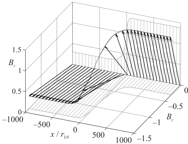
Рис. 2. (Цветной онлайн) Токовый слой с широким диапазоном силовых линий магнитного поля (черные прямые), составленный из двух слоев с планарными полями B_z(x) и B_y(x) \approx -B_z(-x) (синие и оранжевые прямые), каждый из которых сформирован электронной и протонной компонентами с распределениями (14). Для обоих слоев P_0 = 0.55 \sum_{\alpha} N_{\alpha} T_{\alpha} , T_i = 2T_e , N_i = N_e и A_{e,i} = 0 . Индукция поля нормирована на величину B_y(0) = (8\pi P_0)^{1/2} , координата x – на гирорадиус теплового электрона в этом поле B_y(0)
