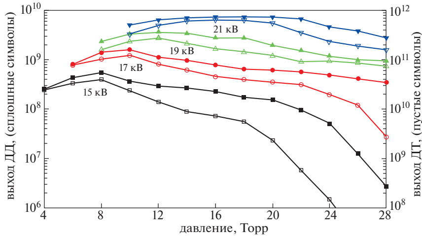
Рис. 3. Нейтронный выход в зависимости от давления для нескольких значений напряжения зарядки.
