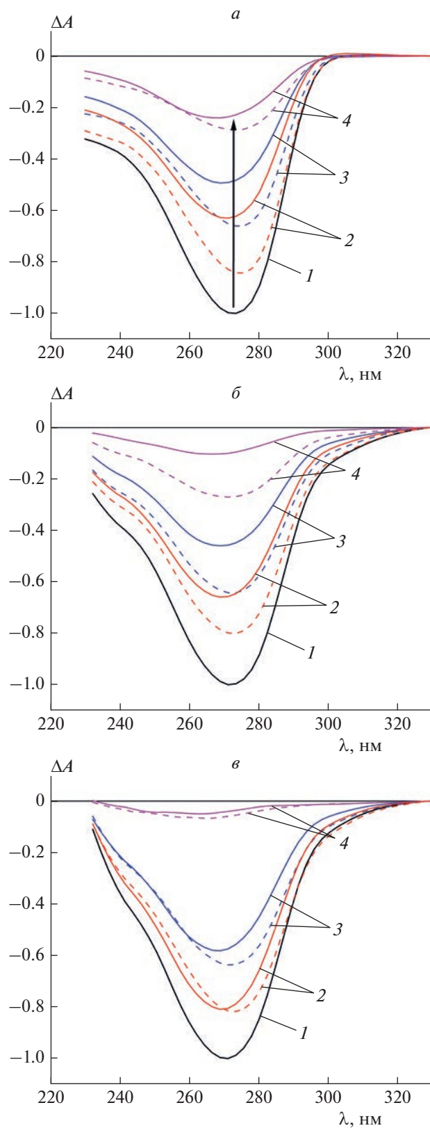
Рис. 3. Нормированные спектры КД трех систем, обработанных НЧЗ: ХЖКД ДНК в отсутствие красителей (а) и в присутствии 7.00 \cdot 10^{-6} М SG (б) или PG (в). Красители и НЧЗ вносили в систему до или после формирования ХЖКД (сплошные и штриховые кривые соответственно). Концентрация НЧЗ составляла 0 (1), 2.27 \cdot 10^{-8} (2), 4.46 \cdot 10^{-8} (3) и 10.55 \cdot 10^{-8} М (4).
