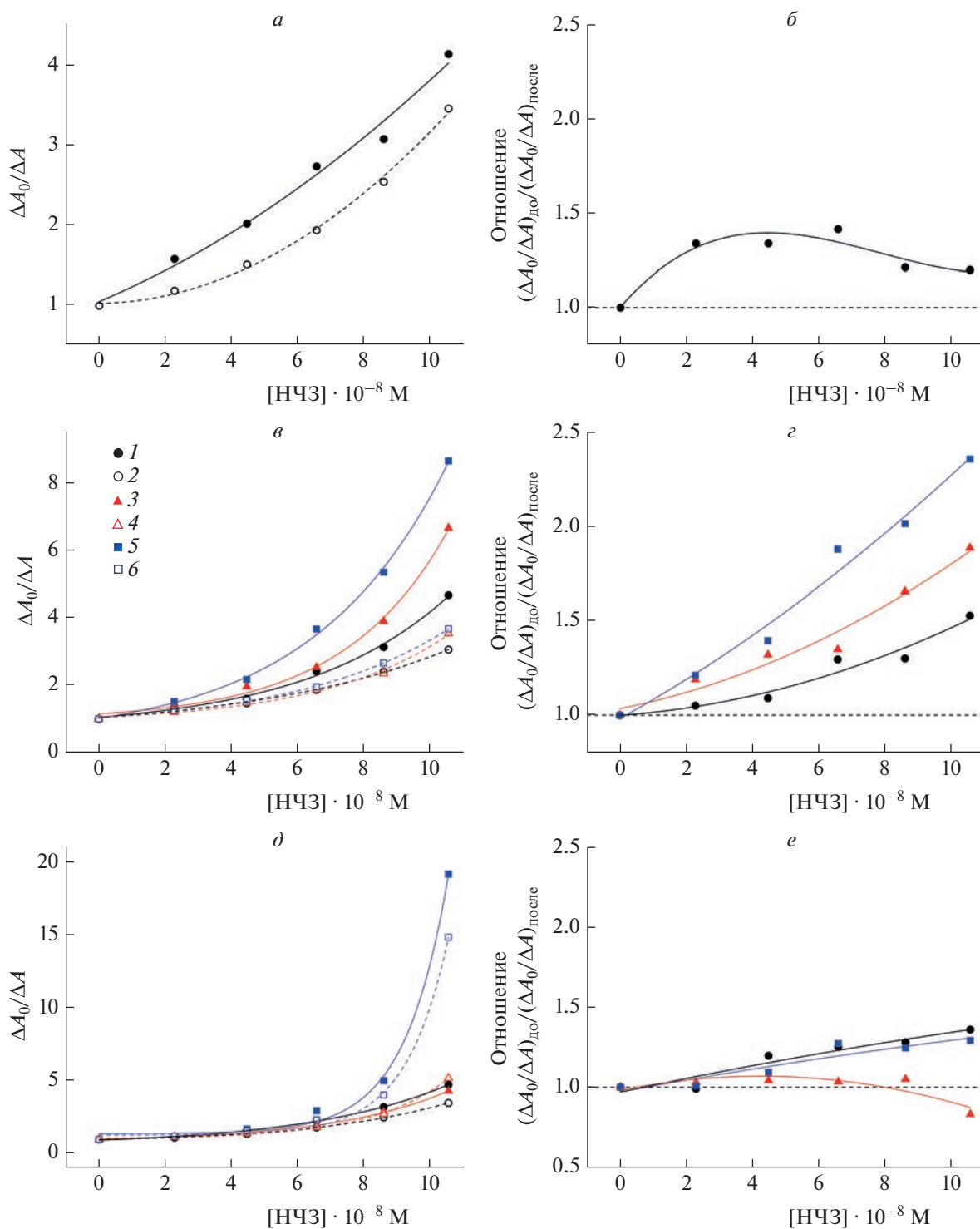
Рис. 4. Разрушение холестерической фазы ДНК под действием НЧЗ в отсутствие ( a ) и в присутствии красителей SG ( б ) или PG ( д ) в концентрации 1.40 \cdot 10^{-6} (●, ○), 3.50 \cdot 10^{-6} (▲, △) и 7.00 \cdot 10^{-6} М (■, □). Сплошные кривые соответствуют предварительной инкубации частиц с ДНК, а штриховые — их введению в готовую дисперсную систему. Отношение степени разрушения холестерической фазы ДНК при разной последовательности введения НЧЗ в систему, не содержащую ( б ) и содержащую красители SG ( з ) или PG ( е ) в концентрации 1.40 \cdot 10^{-6} (●), 3.50 \cdot 10^{-6} (▲) и 7.00 \cdot 10^{-6} М (■). Стандартные отклонения, рассчитанные по трем независимым измерениям, не превышали 8% ( a , в , д ) и 11% ( б , з , е ) соответственно.
