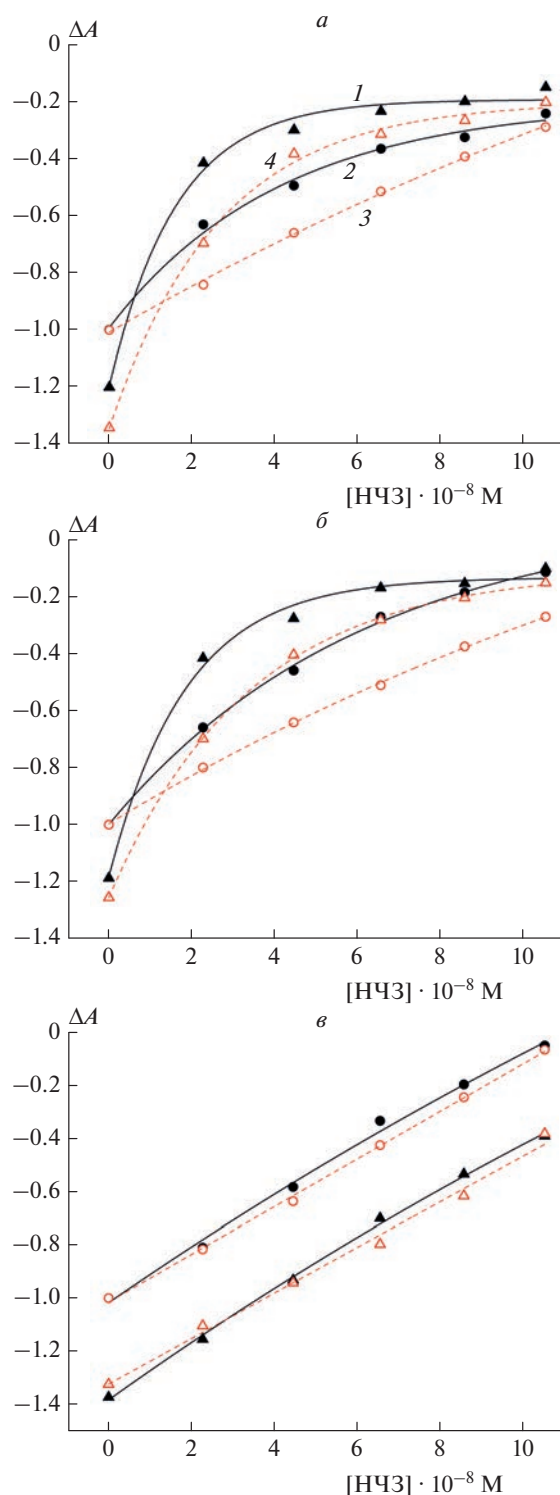
Рис. 5. Зависимости нормированной на начальное значение амплитуды КД-сигнала ХЖКД ДНК от концентрации НЧЗ до тепловой обработки (● и ○) и после цикла нагрев–охлаждение 20°C → 80°C → 20°C (▲ и △) в отсутствие красителей (а) и в присутствии 7.00 \cdot 10^{-6} M SG (б) или PG (в). Кривые с маркерами ● и ▲ соответствуют предварительной инкубации красителей и НЧЗ с ДНК, а с маркерами ○ и △ – их внесению в готовую дисперсную систему. Стандартные отклонения, рассчитанные по трем независимым измерениям, не превышали 5%.
