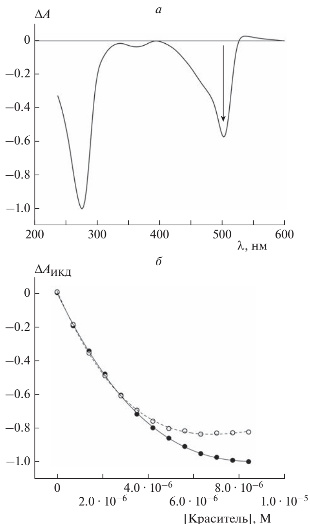
Рис. 2. а – КД-спектр ХЖКД ДНК в присутствии 4.90 \cdot 10^{-6} М красителя PG, нормированный на величину сигнала на длине волны \lambda = 275 нм; б – зависимость интенсивности сигнала ИКД, нормированной на минимальное значение амплитуды индуцированной полосы, от концентрации красителей SG (●) и PG (○). Стандартные отклонения, рассчитанные по трем независимым измерениям, не превышали 5%.
