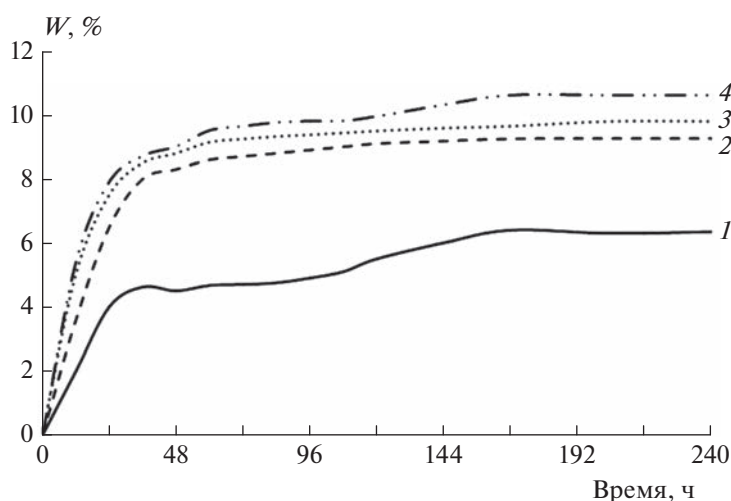
Рис. 4. Зависимость степени водопоглощения ( W ) от содержания термически состаренного ПЭНП, мас. %: 1 – 30 ПЛА/70 ПЭНП, 2 – 30 ПЛА/40 ПЭНП/30 ПЭНПс, 3 – 30 ПЛА/30 ПЭНП/40 ПЭНПс, 4 – 30 ПЛА/20 ПЭНП/50 ПЭНПс.
