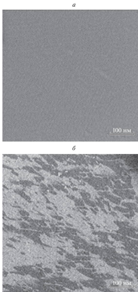
Рис. 1. Микрофотографии СЭМ образцов пленок ПЛА/ПЭНП, мас. %: а — 100/0 (увеличение 215×), б — 30/70 (увеличение 215×).
