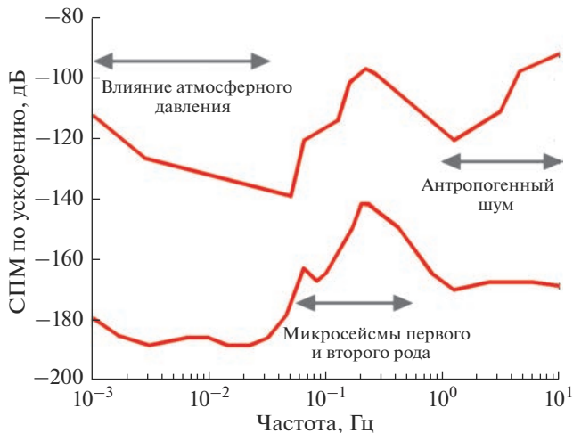
Рис. 1. Минимальный и максимальный уровень микросейсмического шума по модели [Peterson, 1993] с отмеченными основными механизмами в соответствующих диапазонах частот.
