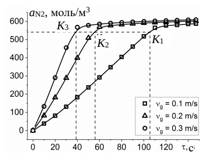
Рис. 1. Кинетические кривые адсорбции азота на цеолитовом адсорбенте NaX: a – при температурах газовой смеси 293, 303, 323 К; б – при давлениях газовой смеси (2, 4, 6)·10 5 Па; в – при скоростях газового потока 0,1; 0,2; 0,3 м/с (точки – эксперимент; линии – расчет; K 1 , K 2 , K 3 – точки разграничения
