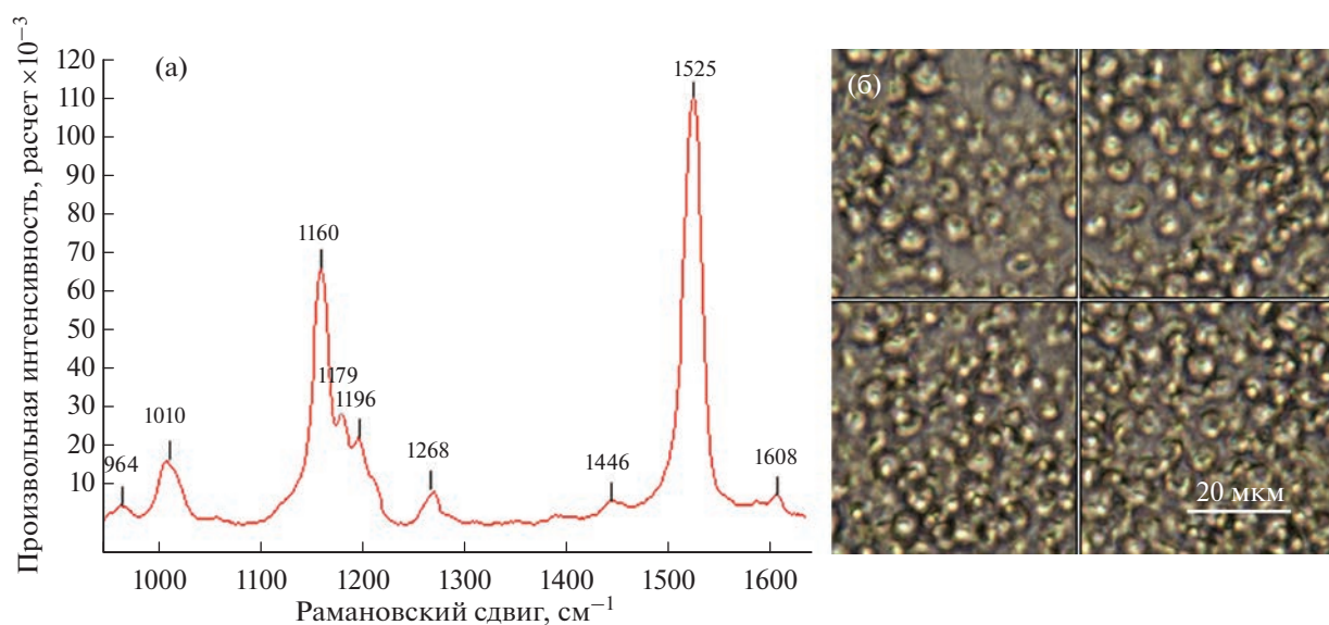
Рис. 5. Рамановский спектр Tisochrysis lutea : а — моды фукоксантина ( \nu_1 1525, \nu_2 1160, \nu_3 1010 \text{cm}^{-1} ); б — точка получения рамановского спектра (клетка).
