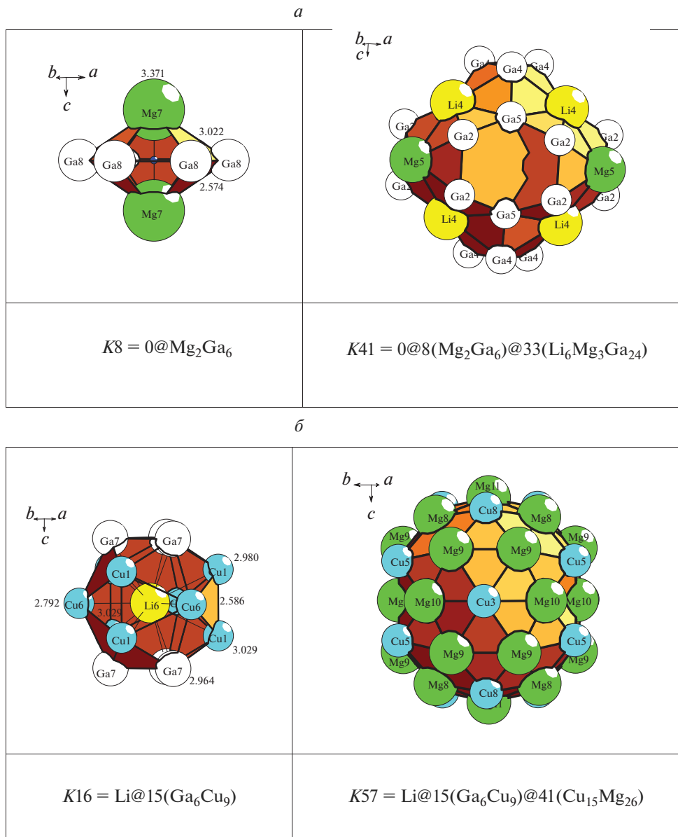
Рис. 1. Li_{10}Mg_{34}Cu_{24}Ga_{71} - hP139 . Кристаллообразующий нанокластер K57 = Li@15(Ga_6Cu_9)@41(Cu_{15}Mg_{26}) с внутренним полиэдром Франка–Каспера Li@15(Ga_6Cu_9) (а) и нанокластер K41 = 0@8(Mg_2Ga_6)@33(Li_6Mg_3Ga_{24}) с внутренним полиэдром в виде гексагональной бипирамиды 0@8(Mg_2Ga_6) (б).
