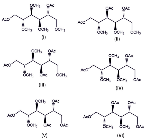
Рис. 5. Перметилованные альдитолацетаты: 1,5-ди- O -ацетил-2,3,4,6-тетра- O -метил-глюцитол (I); 1,3,5-три- O -ацетил-2,4,6-три- O -метил-глюцитол (II); 1,4,5-три- O -ацетил-2,3,6-три- O -метил-глюцитол (III); 1,5,6-три- O -ацетил-2,3,4-три- O -метилглюцитол (IV); 1,4,5,6-тетра- O -ацетил-2,3-ди- O -метилглюцитол (V); 1,3,5,6-тетра- O -ацетил-2,4-ди- O -метил-глюцитол (VI).
