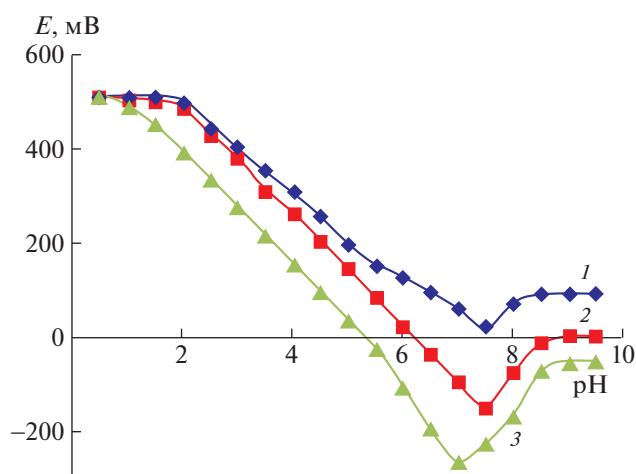
Рис. 1. Зависимости ЭДС ( E , мВ) от рН для системы Fe(II)–Fe(III)–H 2 Sal–C 2 H 5 OH–H 2 O при температуре 298.16 К, ионной силе раствора 1.0 моль/л и различных концентрациях (моль/л): C_{\text{Fe(III)}} = 1 \times 10^{-4} (1), 1 \times 10^{-3} (2, 3); C_{\text{Fe(II)}} = 1 \times 10^{-4} (1), 1 \times 10^{-3} (2, 3); C_L = 1 \times 10^{-3} (1), 1 \times 10^{-2} (2), 5 \times 10^{-2} (3).
