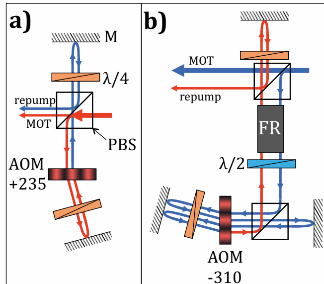
Рис. 5. Оптическая схема добавления частоты перенакачки («гермп») к основной частоте магнитооптического пленения («МОТ»): a — для ^{39}\text{K} ; b — для ^{40}\text{K} . Лучи, нарисованные близко и параллельно, находятся в одной пространственной моде, в том числе лучи «МОТ» и «гермп». «AOM+235» и «AOM-310» — АОМы, сдвигающие частоту света на +235 и -310 МГц соответственно. «PBS» — поляризирующая делительная пластина; « \lambda/2 » и « \lambda/4 » — полу- и четвертьволновой фазовращатель соответственно; «FR» — фарадеевский вращатель поляризации на 45^\circ ; «M» — зеркало
