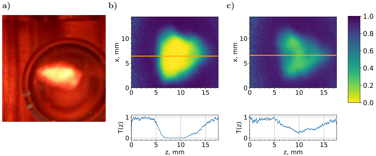
Рис. 6. a — Флуоресценция нескольких миллиардов атомов ^{39}\text{K} в МОЛ. b, c — Теневые снимки для облака ^{39}\text{K} без разлета при отстройке подсвечивающего луча \Delta_{\text{photo}} = -0.2\text{Г} ( b ) и \Delta_{\text{photo}} = 2.5\text{Г} ( c ). Показано распределение коэффициента пропускания T(x, z) , величина которого отражена в цвете. Под каждым снимком показано распределение T(x = \text{const}, z) вдоль оранжевой линии, сглаженное по соседним точкам вдоль линии. На панели ( c ) видимое число атомов N = 8.7 \cdot 10^9
