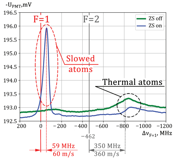
Рис. 4. Флюоресценция пучка атомов, прошедших через зеemanовский замедлитель, в зависимости от \Delta\nu_{F=1} , отстройки диагностического луча от частоты перехода 4S_{1/2}(F = 1) \rightarrow 4P_{3/2}(F' = 2) . Резонанс с этим переходом и с 4S_{1/2}(F = 2) \rightarrow 4P_{3/2}(F' = 3) отмечен вертикальными линиями «F = 1» и «F = 2» соответственно. «ZS on/off» — замедлитель включен/выключен. Флюоресценция измерена в единицах выходного напряжения ФЭУ U_{\text{РМТ}} и видна на фоне засветки ФЭУ переотражениями
