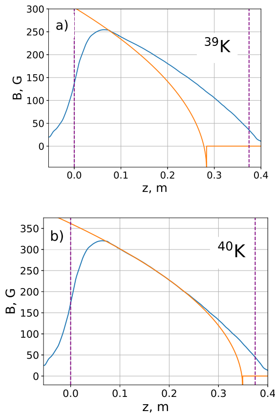
Рис. 3. Профиль магнитного поля на оси зеemanовского замедлителя для ^{39}\text{K} (a) и ^{40}\text{K} (b). Синим — измеренное поле при 7.7 А (a, для ^{39}\text{K} ) и 9.7 А (b, для ^{40}\text{K} ), оранжевым — поле идеального замедлителя (1) для заданных отстроек \Delta_0 . Вертикальными штриховыми линиями показаны границы электромагнита
