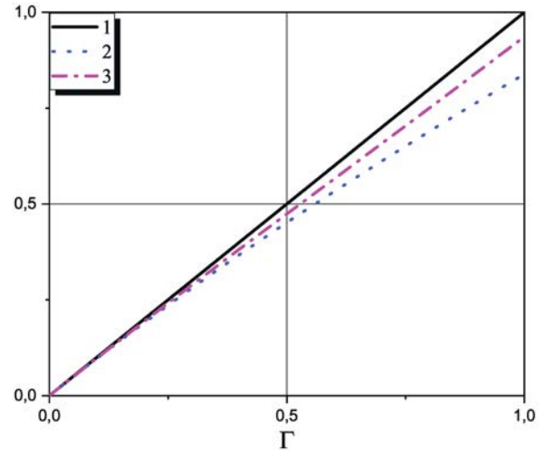
Рис. 1. Решение уравнения Ликальтера \alpha(\Gamma) для \delta = 2 : 1 — \Gamma ; 2 — EL-модель, уравнение (16); 3 — VKS-модель, уравнение (32)
