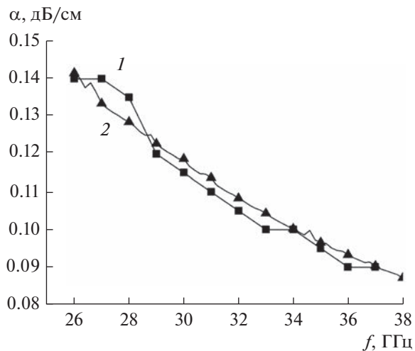
Рис. 5. Зависимость погонных потерь \alpha от частоты f в диэлектрическом волноводе для E_{11}^y : 1 — эксперимент, 2 — расчет.
