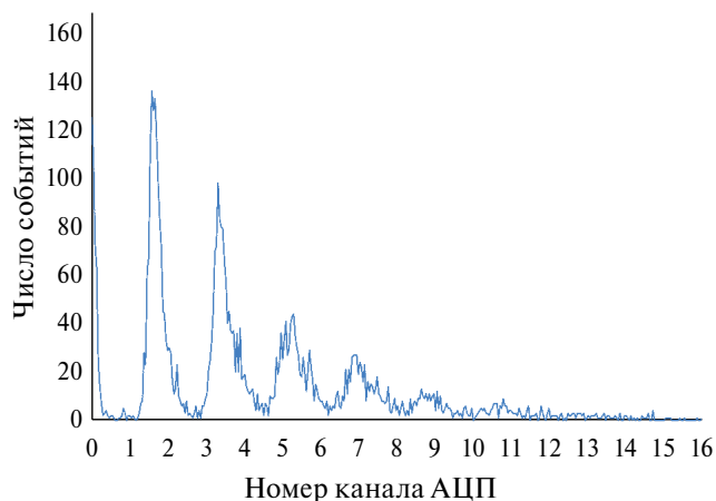
Рис. 13. Калибровочный спектр при малом количестве фотоэлектронов. Левый пик в спектре соответствует педесталу, последующие — импульсам однофотонных сигналов, двухфотонных и так далее.
