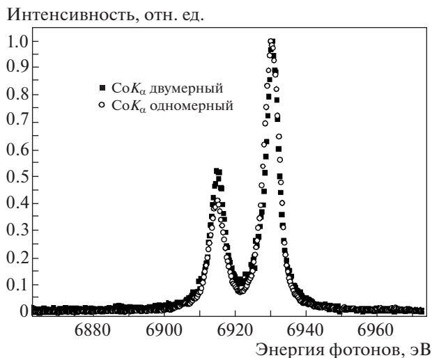
Рис. 5. Сравнение \text{CoK}_{\alpha} -спектров, полученных с помощью одномерного позиционного и двумерного детекторов.
