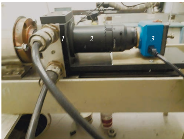
Рис. 1. Система регистрации. 1 – детектор в диэлектрическом кожухе, 2 – объектив TAMRON, 3 – цифровая видеокамера BMR-1400NM-U.
