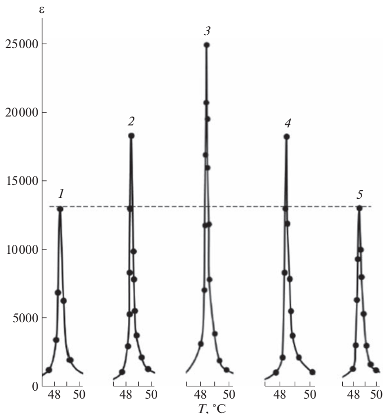
Рис. 1. Эволюция зависимости \epsilon(T) , наблюдаемая в кристалле TGS-Cr-2 вблизи фазового перехода после воздействия магнитного поля: 1 – исходная зависимость \epsilon(T) ; 2, 3, 4, 5 – через 4, 10, 49 и 500 ч после магнитного экспонирования (измерения выполнены при охлаждении образца).
