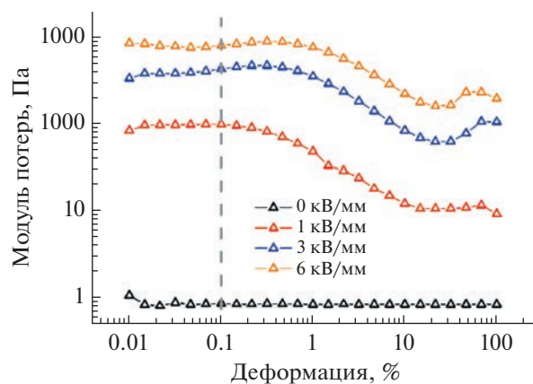
Рис. 5. Зависимость модуля потерь ( G'' ) от деформации для 1 мас. % суспензии МКЦ в оливковом масле при различной напряженности электрического поля, частота измерений 10 Гц. Серой пунктирной линией отмечена величина деформации, далее используемая для нахождения частотных зависимостей модулей накопления и потерь.
