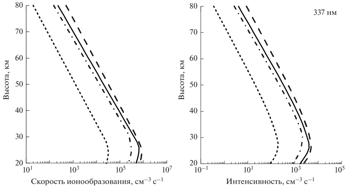
Рис. 2. Профили рассчитанных скоростей ионизации и скоростей объемной интенсивности полосы 337 нм молекулярного азота: GLE65 (короткие штрихи), GLE67 (штрихпунктирные линии), GLE69 (длинные штрихи), GLE70 (сплошные линии).
