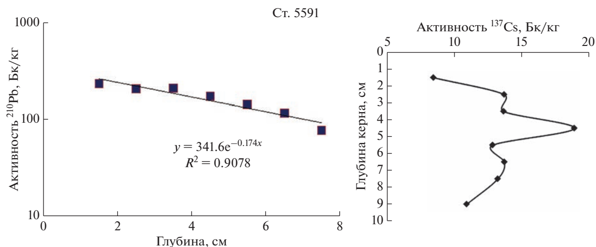
Рис. 2. Изменение удельных активностей избыточного ^{210}\text{Pb} и ^{137}\text{Cs} по глубине колонки 5591.
