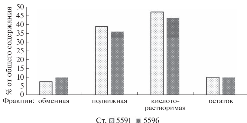
Рис. 4. Формы нахождения ^{239}\text{Pu} в образцах донных отложений моря Лаптевых, % от общего содержания в образце, оцененные по методу (Павлючкая и др., 2003).
