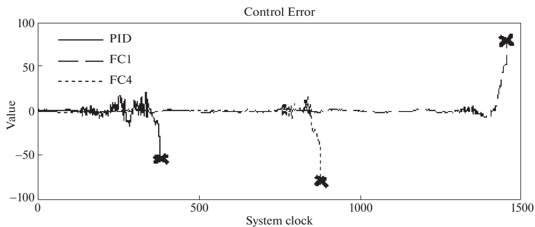
Рис. 21. Угол отклонения макета. Нештатная ситуация управления. Эксперимент
