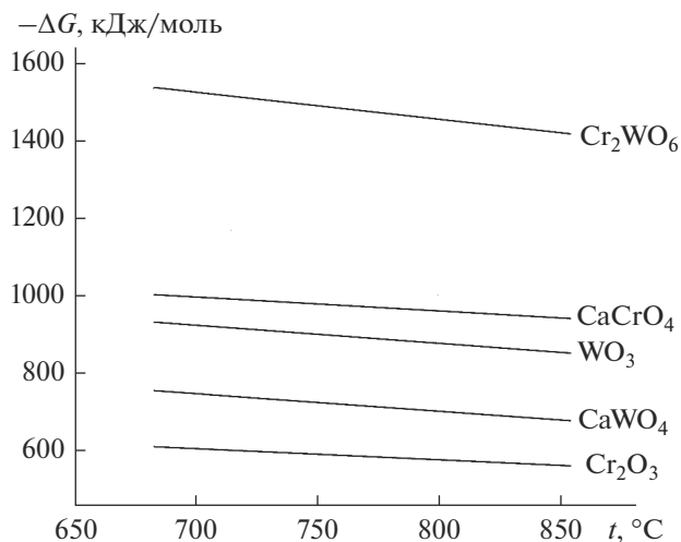
Рис. 2. Зависимости энергии Гиббса \Delta G от температуры реакций восстановления оксидных соединений вольфрама и хрома парами магния.
